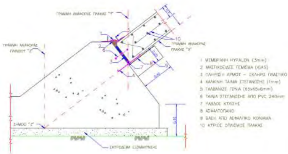
Σχ. 7: Περιμετρικός αρμός
