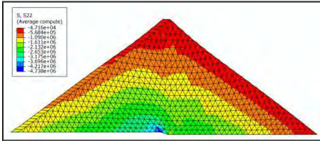
Σχ. 46: Μεταβολή κατακόρυφης ορθής τάσης S_{22}
