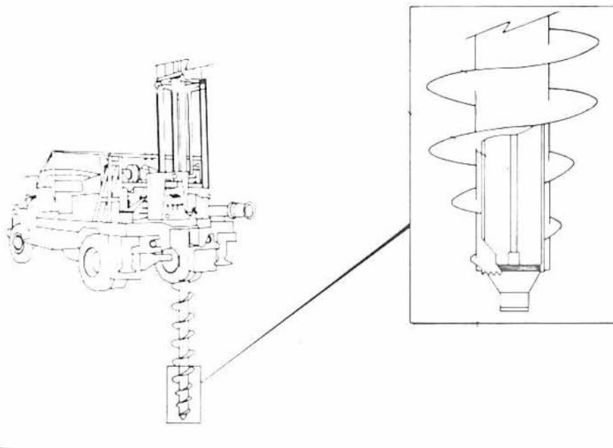
Εικόνα 4.7 Περιστροφικό γεωτρήσιμο.[3]
