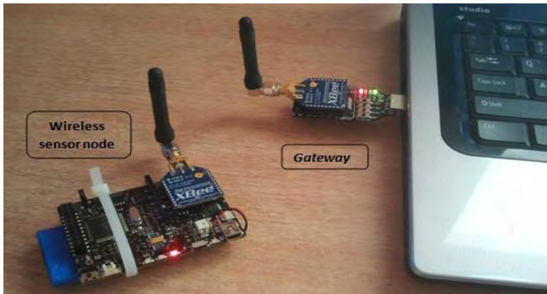
Εικόνα 3-12 : Gateway και ασύρματος κόμβος αισθητήρων
