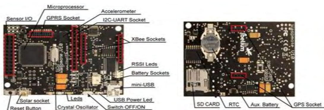
Εικόνα 3-9 : Περιγραφή της βασικής πλακέτας Waspote [17]
