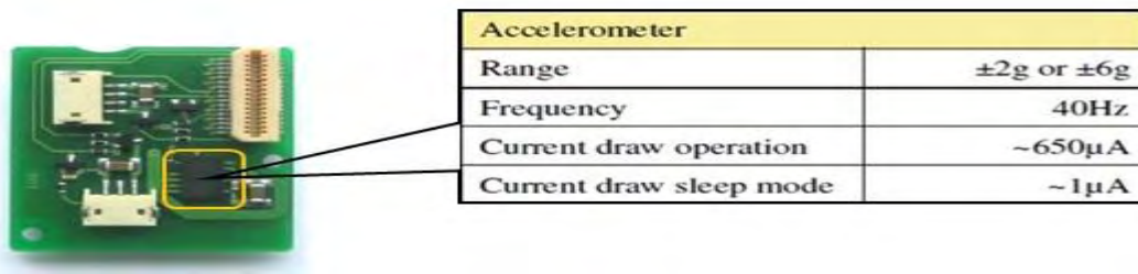
Εικόνα 3-17 : Αισθητήρας επιτάχυνσης του Security Sensor Module
