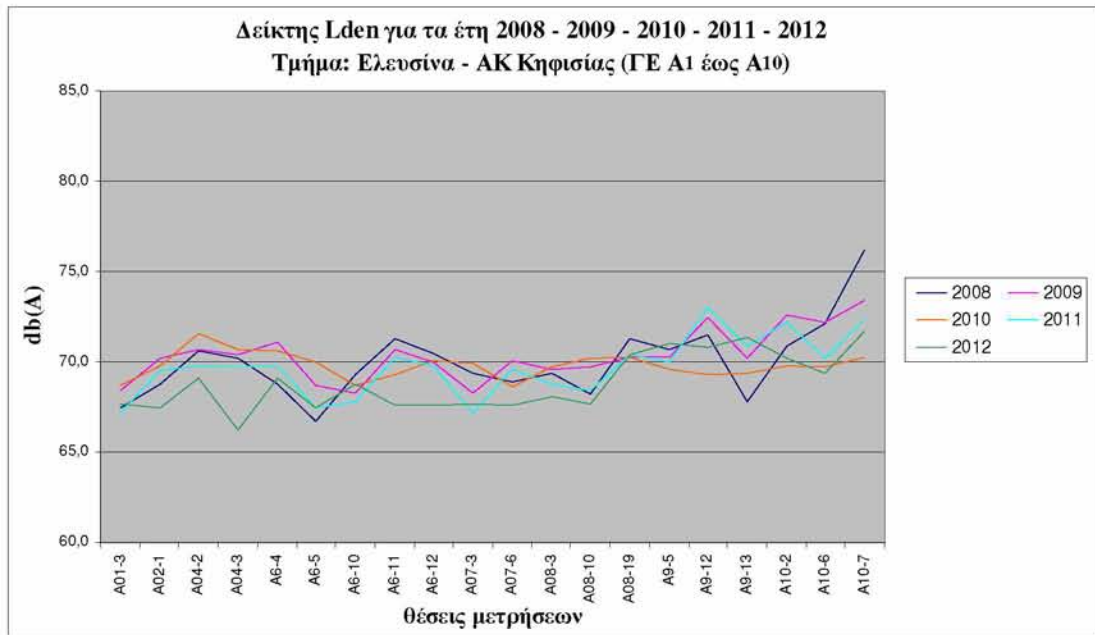
Διάγραμμα 7.6: Κατανομές δείκτη θορύβου Lden για τα έτη 2008,2009,2010,2011,2012 – Τμήμα: Ελευσίνα – ΑΚ Κηφισίας
