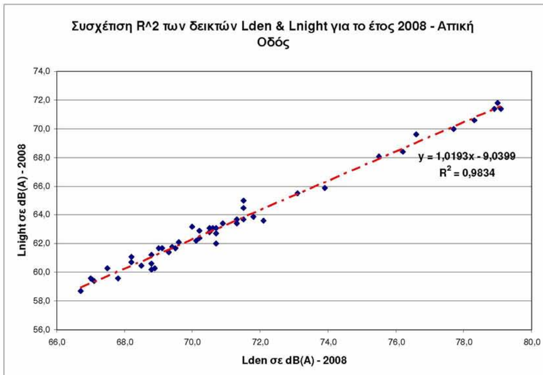
Διάγραμμα 6.9: Συσχέτιση R^2 των δεικτών L_{den} & L_n για το έτος 2008
