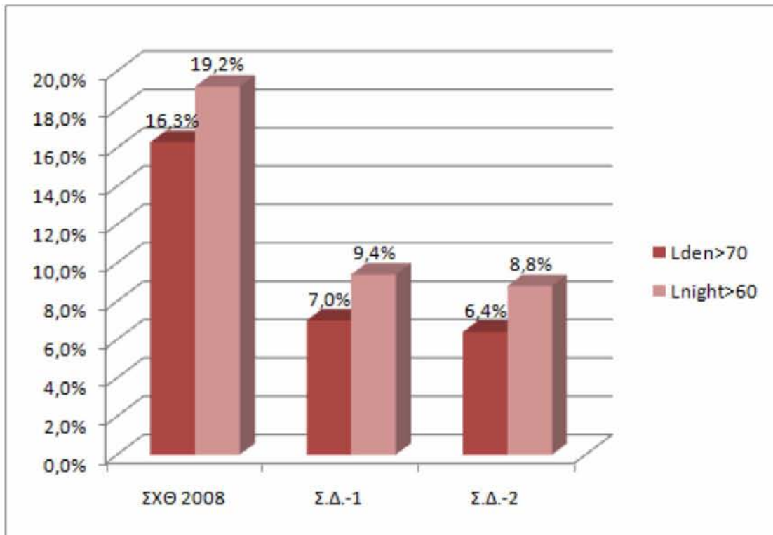
Σχήμα 5.10: Συγκριτική διαφοροποίηση της ποσοστιαίας έκθεσης του πληθυσμού για τις στάθμες Lden>70 dB(A) και Ln night >60 dB(A) για το σύνολο των σεναρίων : ΣΧΘ 2008 (χωρίς αντιθρομβική προστασία και Σχέδια Δράσης ΣΔ-1 και ΣΔ-2
