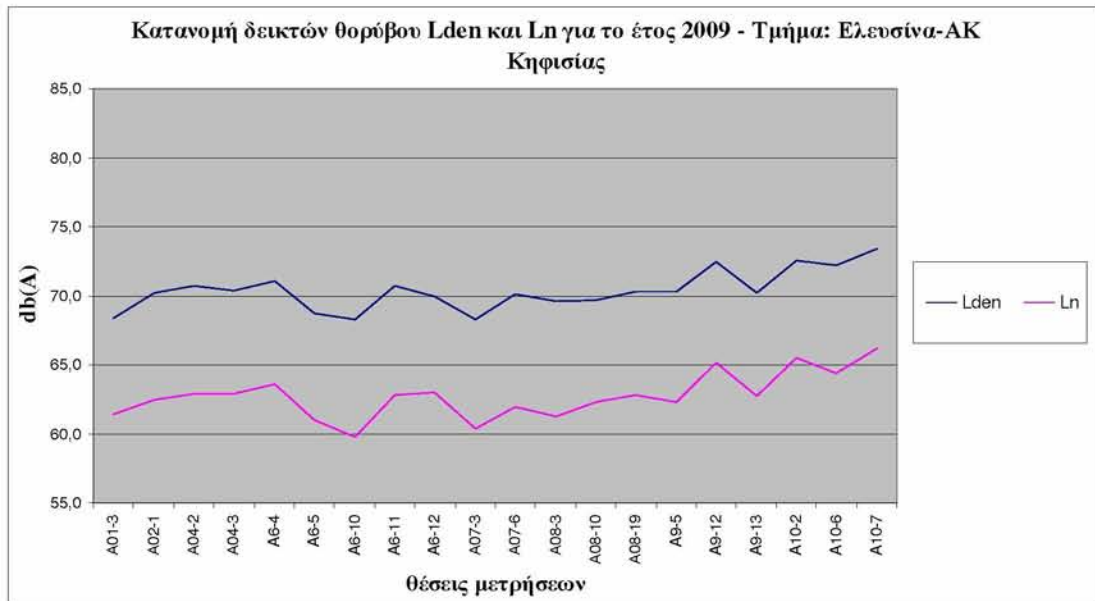
Διάγραμμα 7.2: Κατανομή δεικτών θορύβου Lden & Ln για το έτος 2009 – Τμήμα: Ελευσίνα-ΑΚ Κηφισίας
