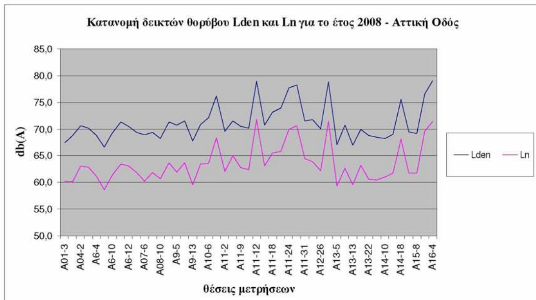
Διάγραμμα 6.1: Κατανομή δεικτών θορύβου Lden & Ln για το έτος 2008
