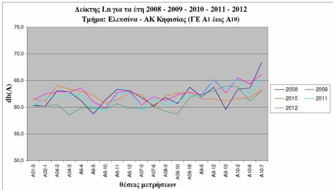
Διάγραμμα 7.7: Κατανομές δείκτη θορύβου Ln για τα έτη 2008,2009,2010,2011,2012 – Τμήμα: Ελευσίνα – ΑΚ Κηφισίας
