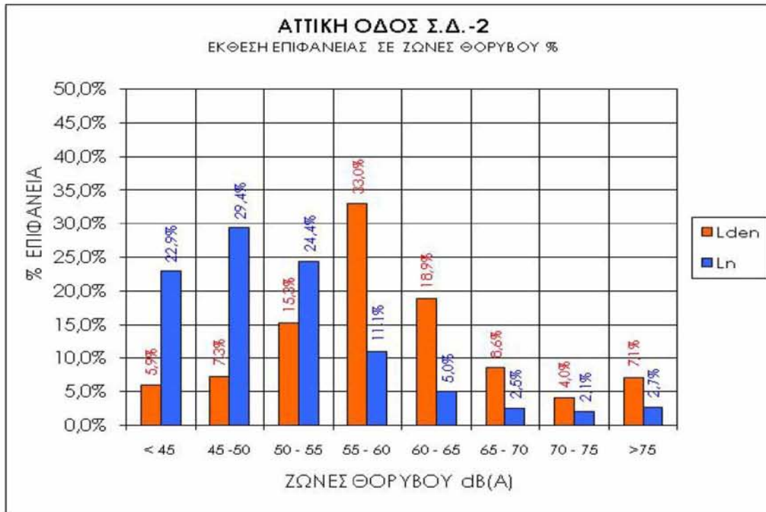
Σχήμα 5.8: Διαγραμματική κατανομή της επιφανείας στις ζώνες των δεικτών οδικού κυκλοφοριακού θορύβου Lden και Ln για το Σχέδιο Δράσης ΣΔ-2 της Αττικής Οδού.
