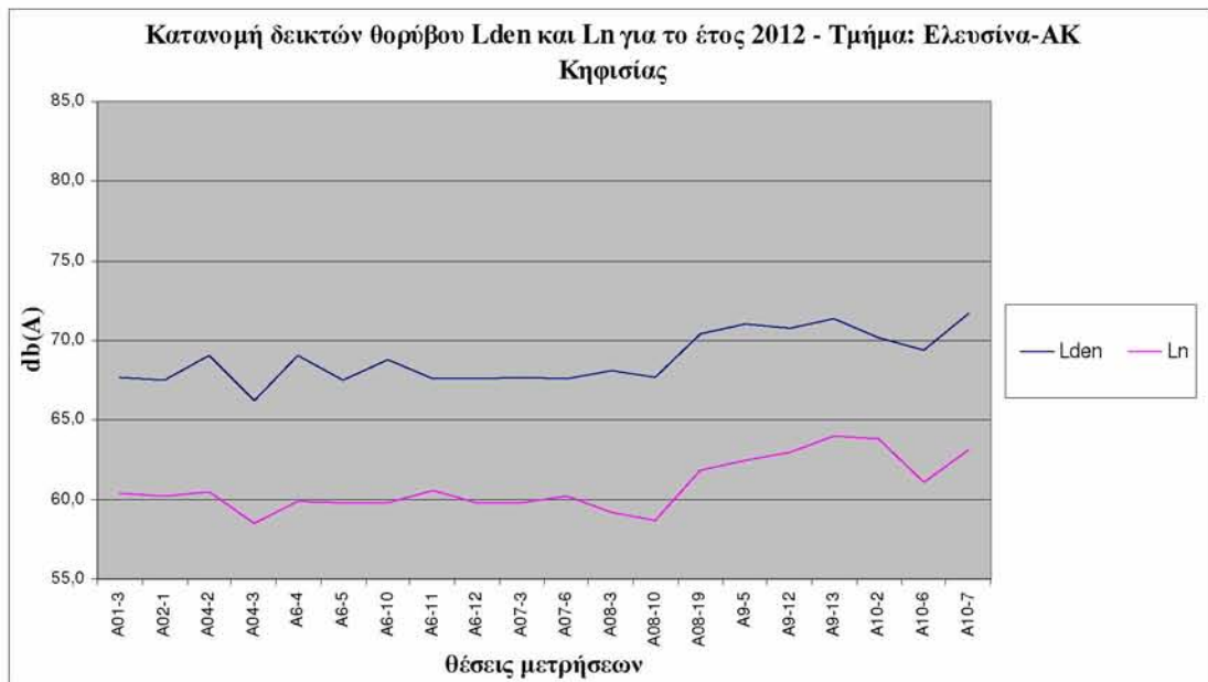
Διάγραμμα 7.5: Κατανομή δεικτών θορύβου Lden & Ln για το έτος 2012 – Τμήμα: Ελευσίνα-ΑΚ Κηφισίας
