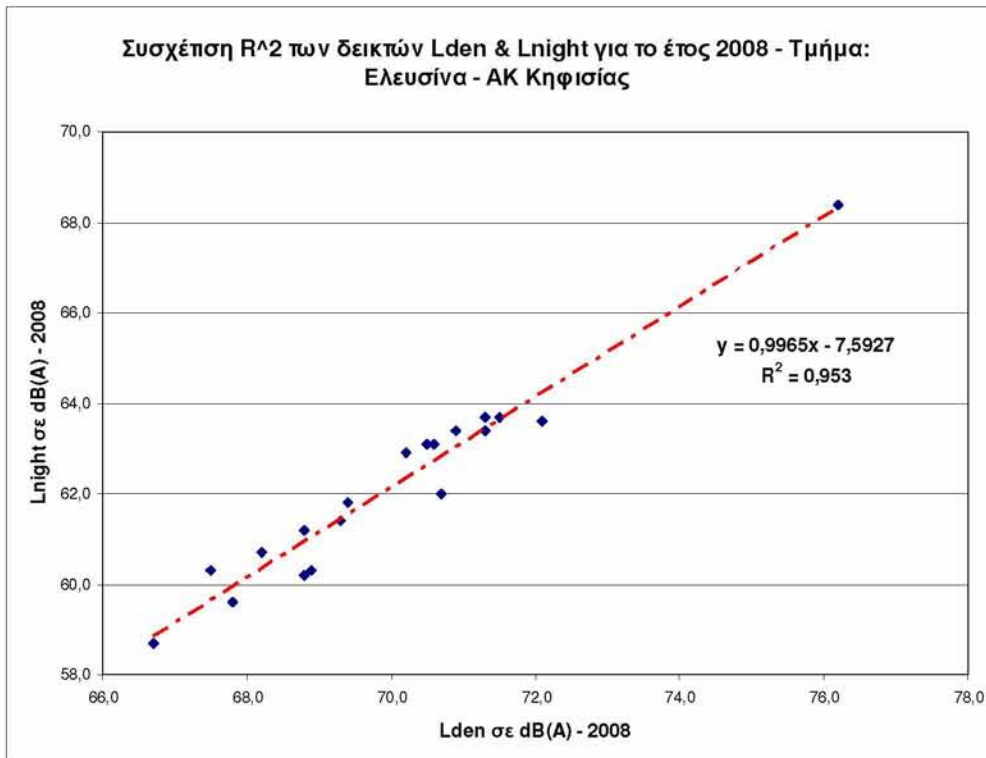
Διάγραμμα 7.9: Συσχέτιση R^2 των δεικτών L_{den} & L_n για το έτος 2008
