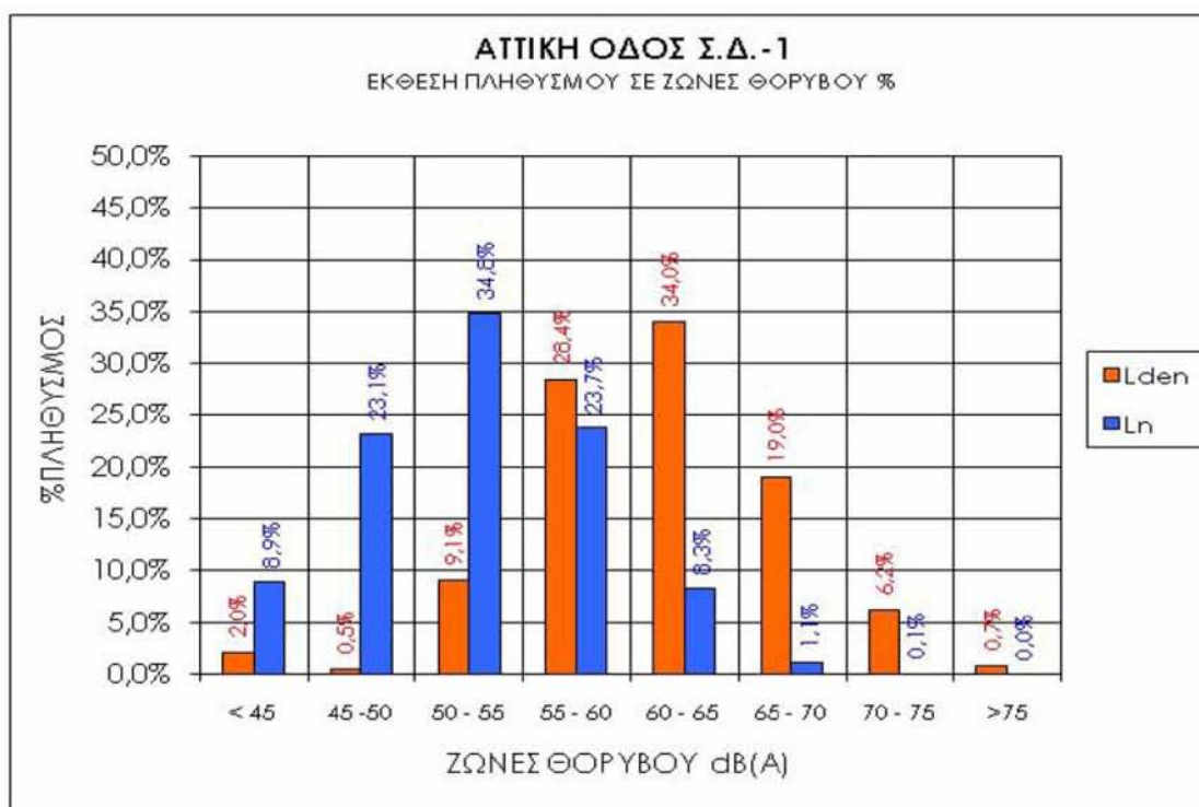
Σχήμα 5.6: Διαγραμματική κατανομή πληθυσμού στις ζώνες των δεικτών οδικού κυκλοφοριακού θορύβου Lden και Lnigh για το Σχέδιο Δράσης ΣΔ-1 της Αττικής Οδού.
