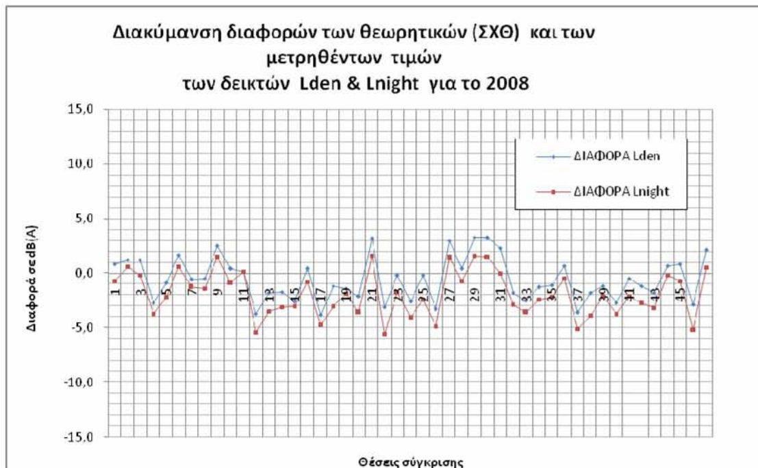
Διάγραμμα 7 19: Διαφορές θεωρητικών και μετρηθέντων τιμών των δεικτών Lden & Ln για το 2008 – 47 σημ
