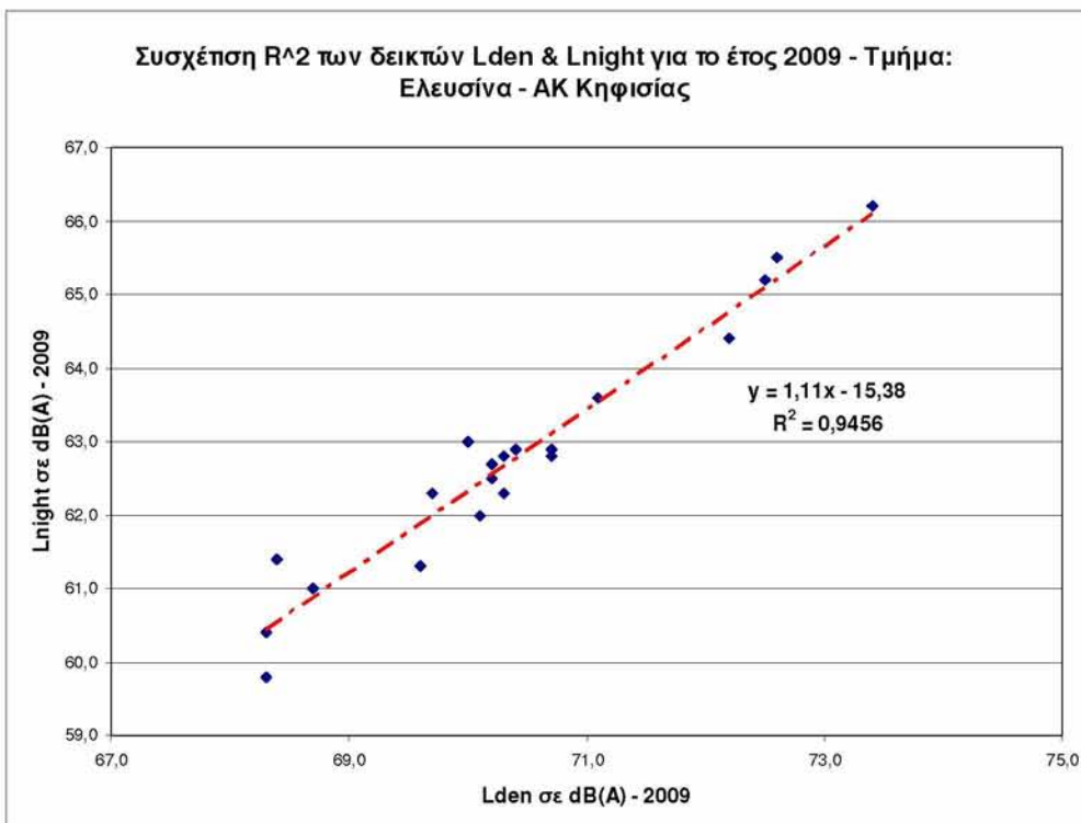
Διάγραμμα 7.10: Συσχέτιση R^2 των δεικτών L_{den} & L_n για το έτος 2009
