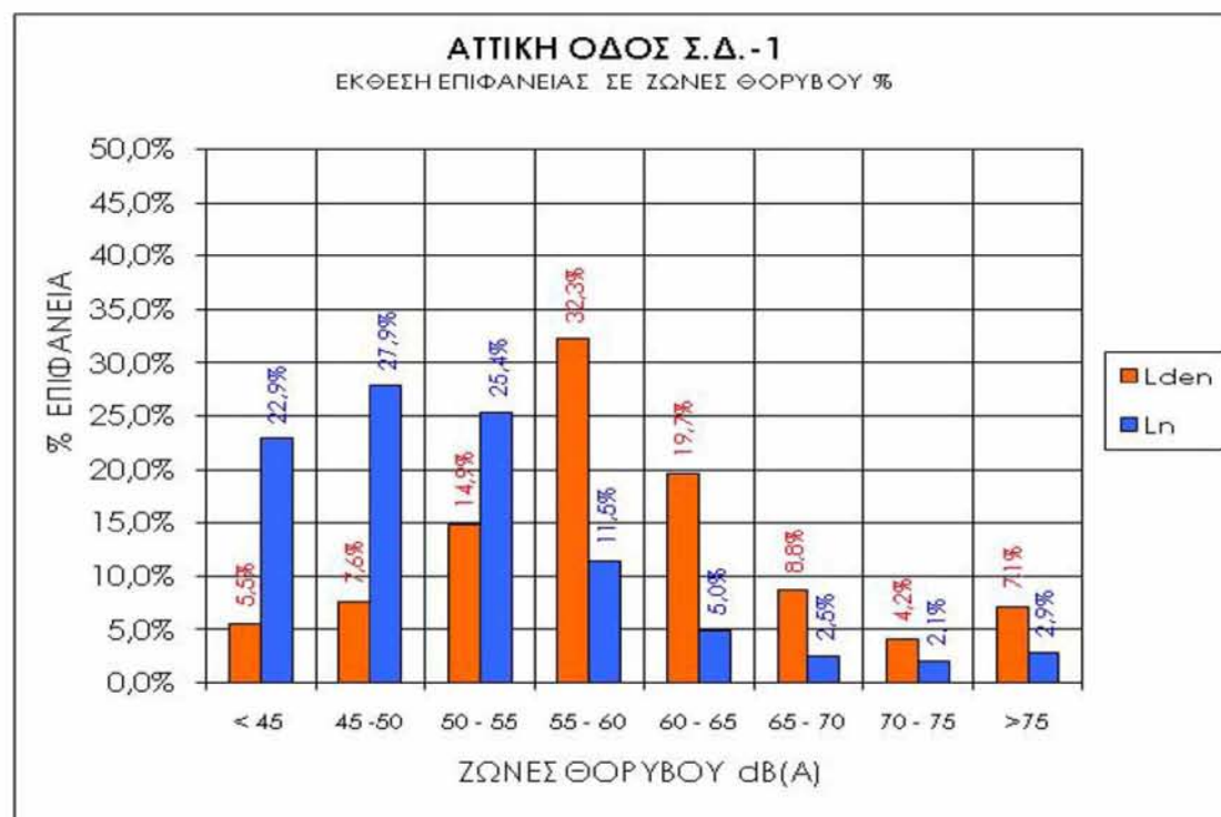
Σχήμα 5.5: Διαγραμματική κατανομή της επιφανείας στις ζώνες των δεικτών οδικού κυκλοφοριακού θορύβου Lden και Lnigh. για το Σχέδιο Δράσης ΣΔ-1 της Αττικής Οδού.
