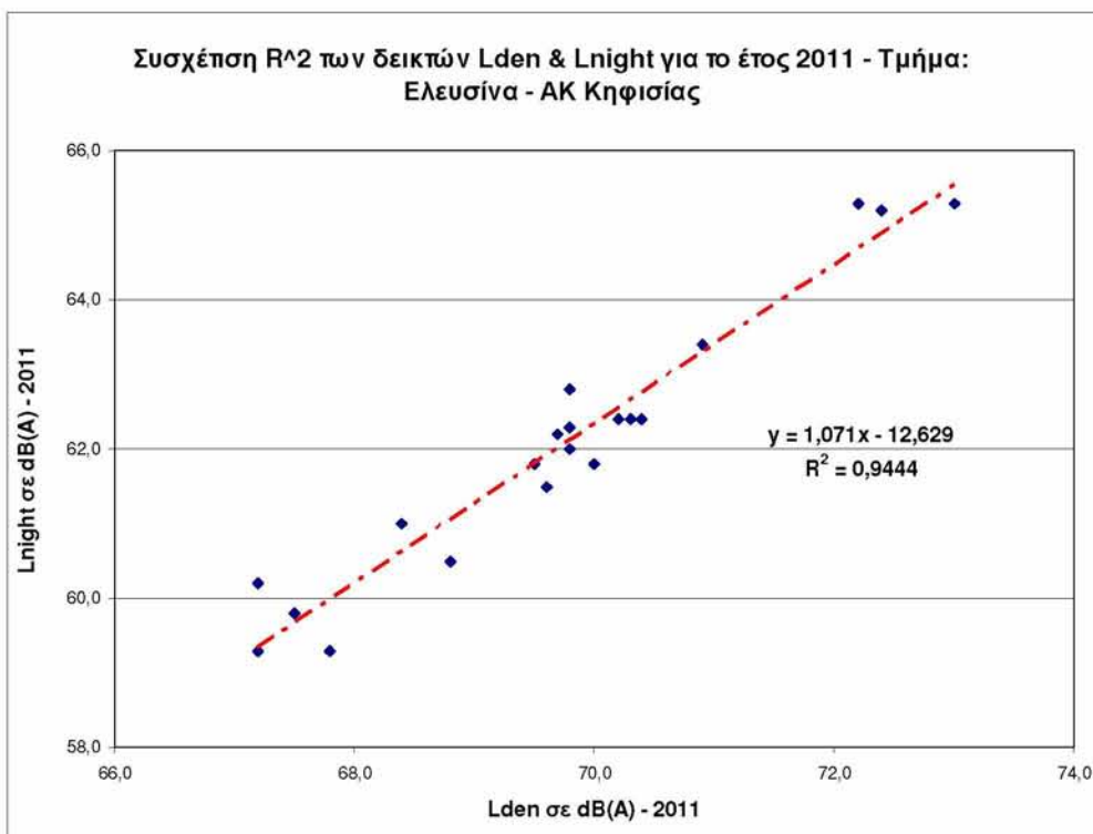
Διάγραμμα 7.12: Συσχέτιση R 2 των δεικτών Lden & Ln για το έτος 2011
