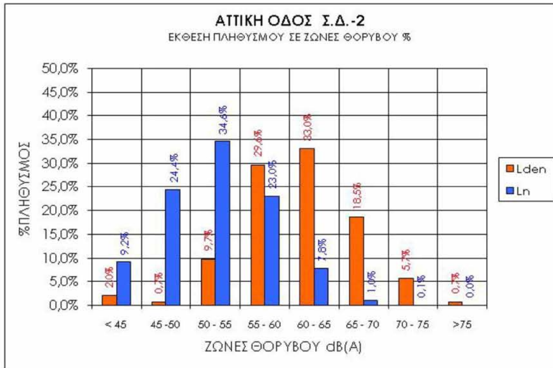
Σχήμα 5.9: Διαγραμματική κατανομή πληθυσμού στις ζώνες των δεικτών οδικού κυκλοφοριακού θορύβου Lden και Ln για το Σχέδιο Δράσης ΣΔ-2 της Αττικής Οδού.
