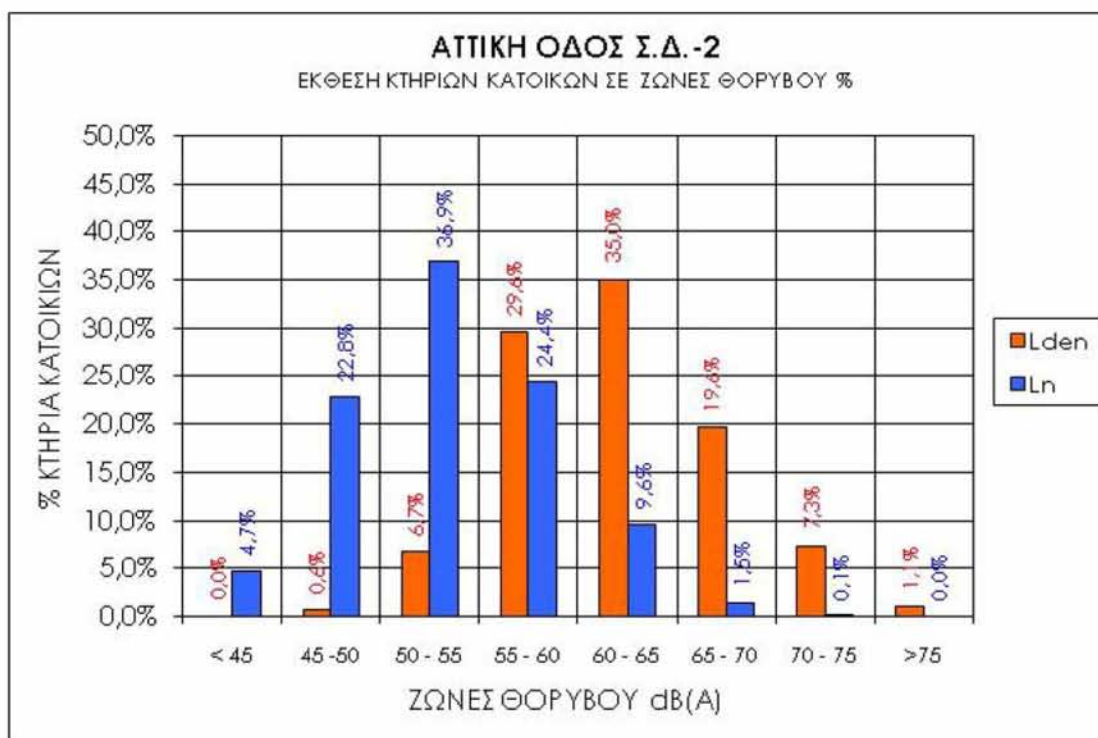
Σχήμα 5.10: Διαγραμματική κατανομή κτηρίων κατοικιών στις ζώνες των δεικτών οδικού κυκλοφοριακού θορύβου Lden και Ln για το Σχέδιο Δράσης ΣΔ-2 της Αττικής Οδού.
