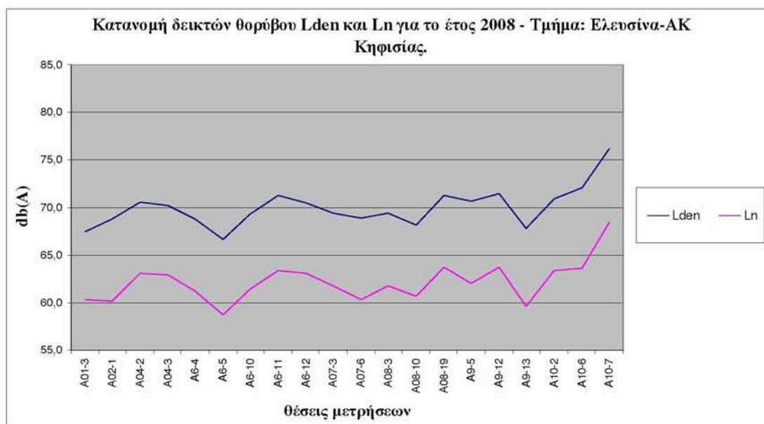
Διάγραμμα 7.1: Κατανομή δεικτών θορύβου Lden & Ln για το έτος 2008 – Τμήμα: Ελευσίνα-ΑΚ Κηφισίας
