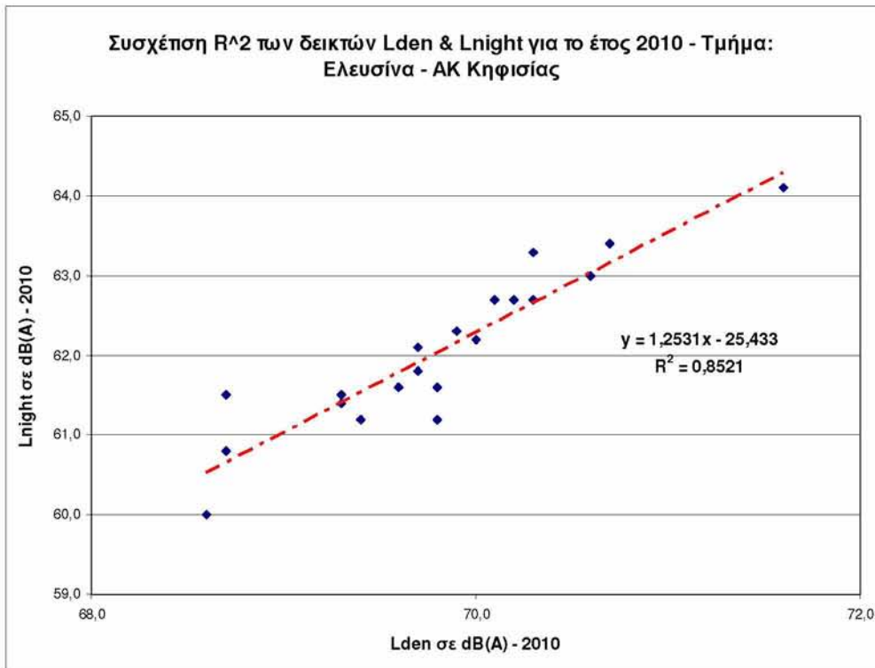
Διάγραμμα 7.11: Συσχέτιση R 2 των δεικτών Lden & Ln για το έτος 2010
