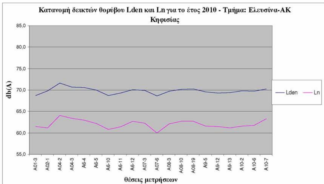
Διάγραμμα 7.3: Κατανομή δεικτών θορύβου Lden & Ln για το έτος 2010 – Τμήμα: Ελευσίνα-ΑΚ Κηφισίας
