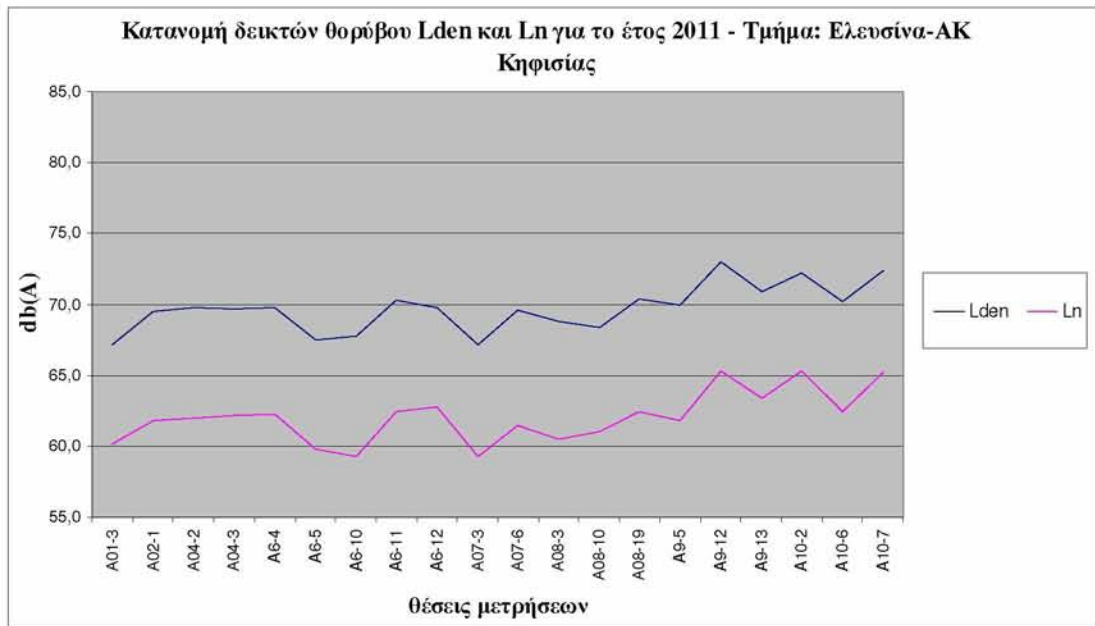
Διάγραμμα 7.4: Κατανομή δεικτών θορύβου Lden & Ln για το έτος 2011 – Τμήμα: Ελευσίνα-ΑΚ Κηφισίας
