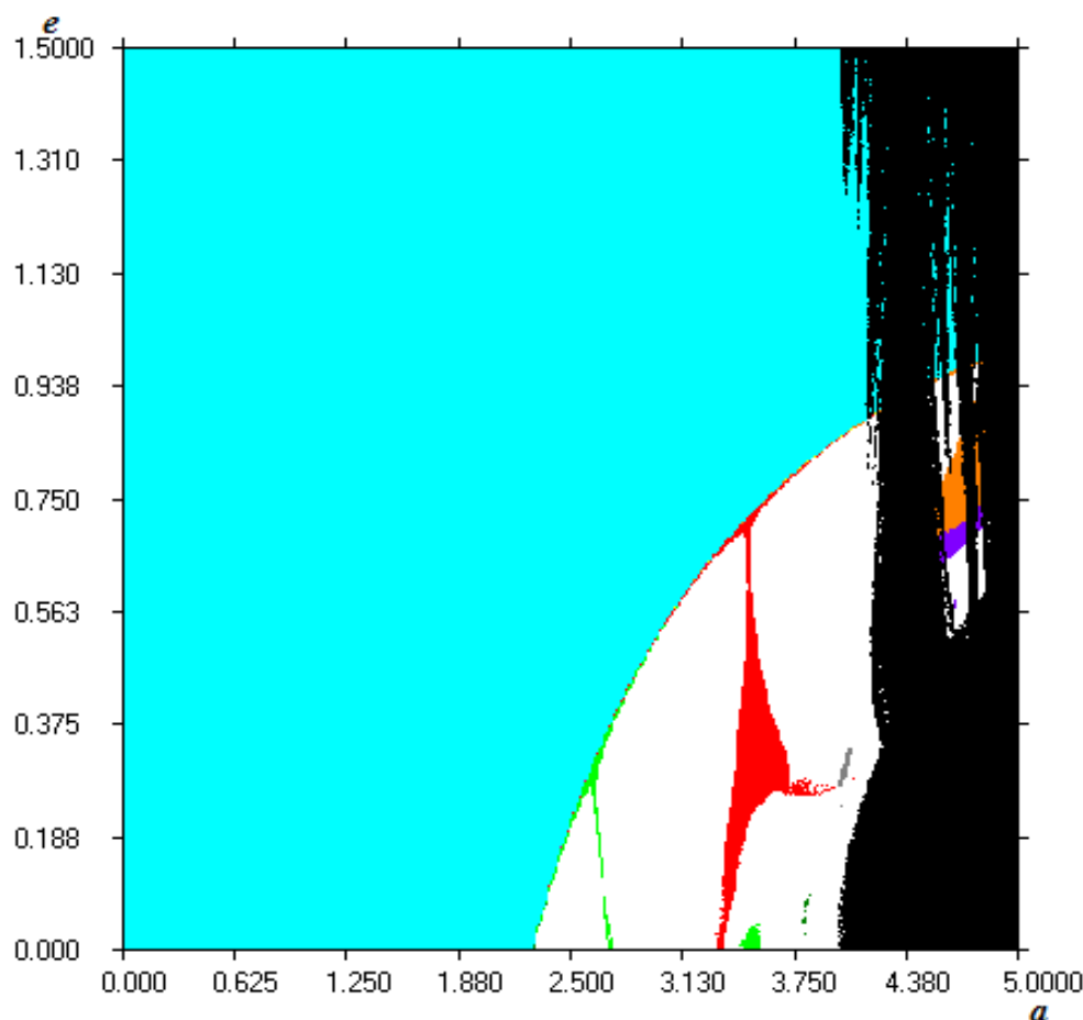
Σχήμα 5.1 Διάγραμμα περιοχών σύγκλισης για \epsilon , a .
