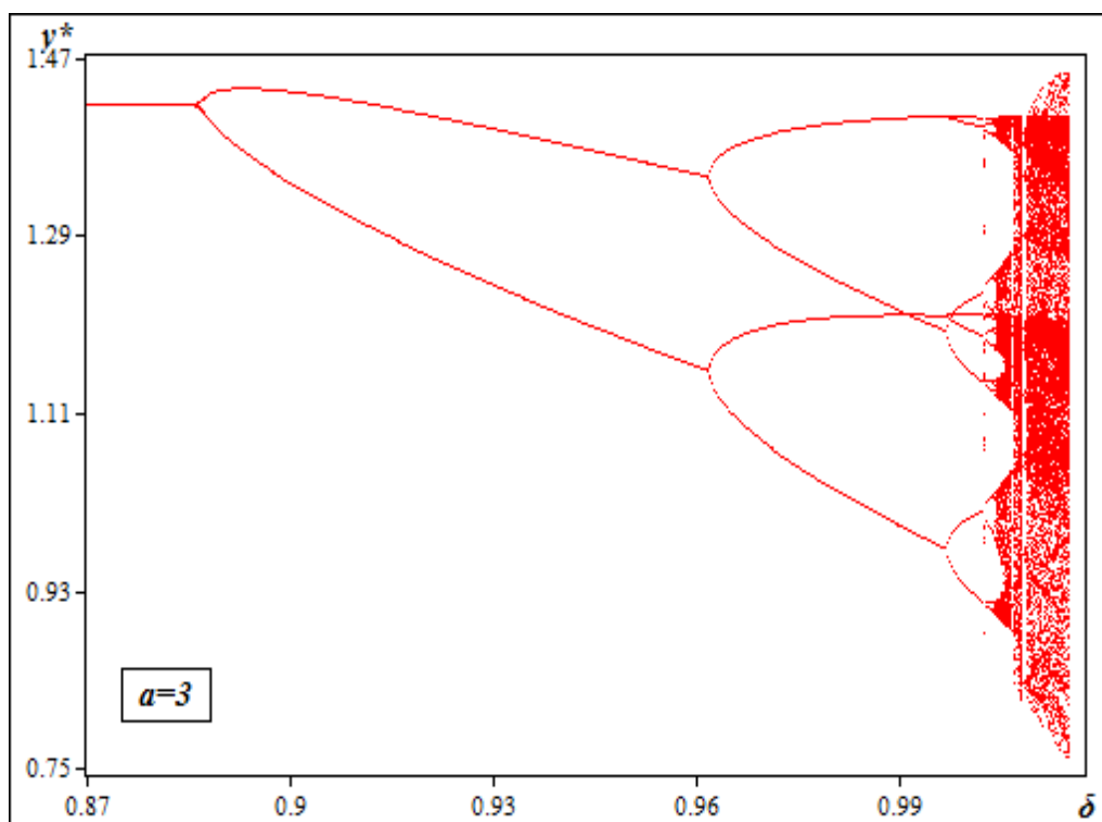
Σχήμα 6.14(γ) Διάγραμμα διακλάδωσης θηρευτή για \alpha = 3 και \delta \rightarrow (0,87 \text{ έως } 1,017)
