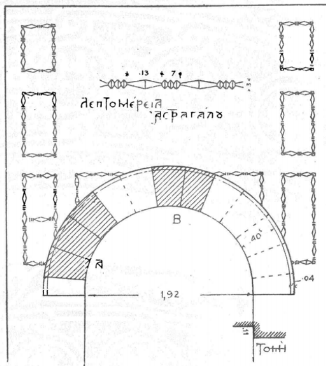
Εἰκ. 53. Διακόσμησης δι' ἀστραγαλιῶν πλαισίων.
