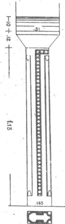
Εἰκ. 10. Πλαγία ὄψις καὶ τομὴ ὁριζοντία τοῦ κιονίσκου τῆς εἰκ. 9.
