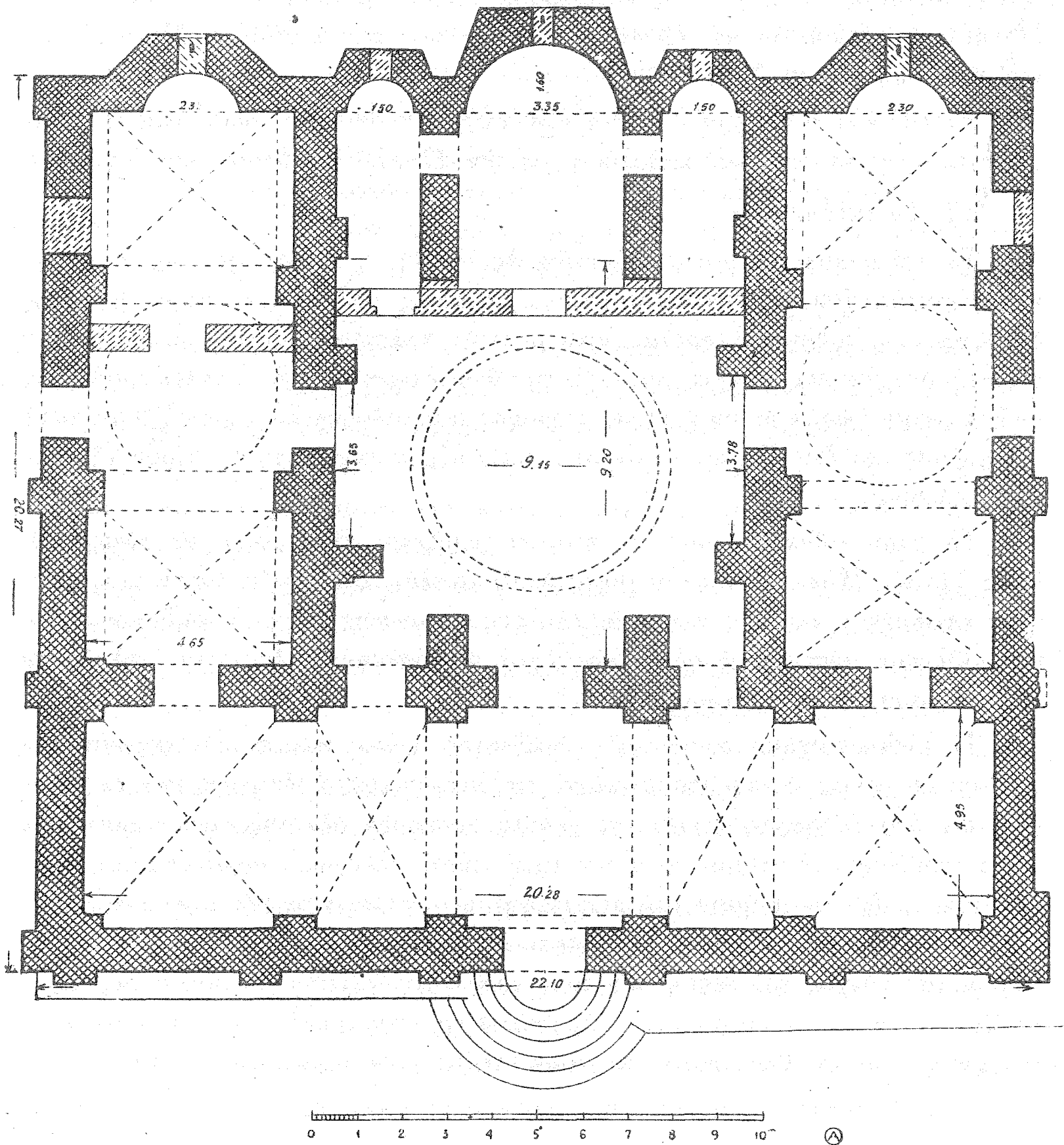
Εἰκ. 3. Κάτοπις τοῦ ἰσογείου.
