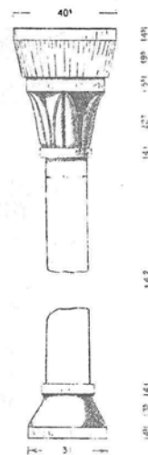
Εἰκ. 17. Ἐσωτερικὸς κιονίσκος τοῦ οὐρανίσκου.
