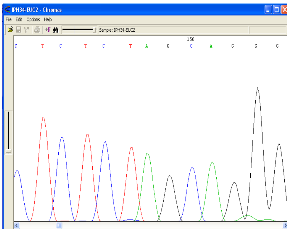
Εικόνα. 26. Μορφή χρωματογραφήματος
