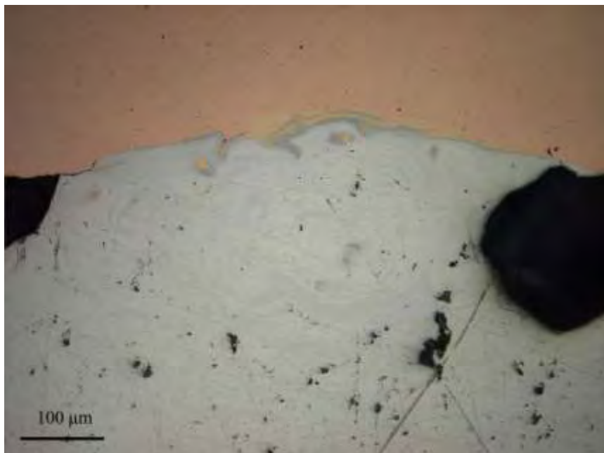
Εικ. 27: Περιοχή συγκόλλησης κατηγορίας A_{new} (200x)
