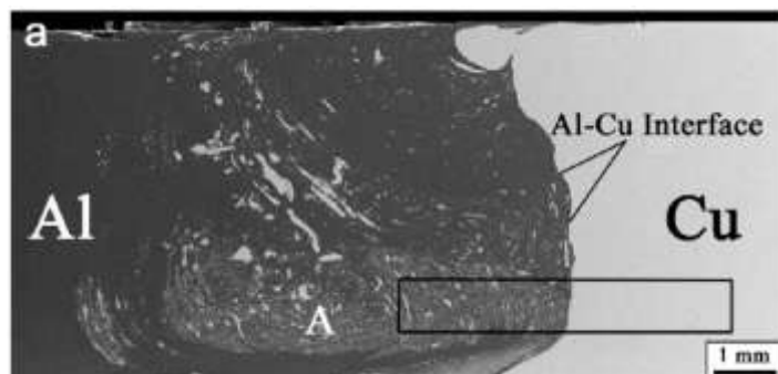
Εικ.2: Μικροδομή SEM (back scatter) από FSW joint [5]
