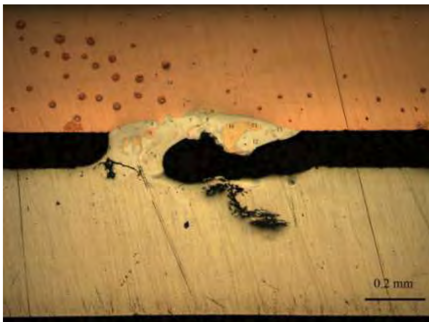
Εικ. 53: Περιοχή συγκόλλησης κατηγορίας A, Σημεία μικροσκληρομετρήσης
