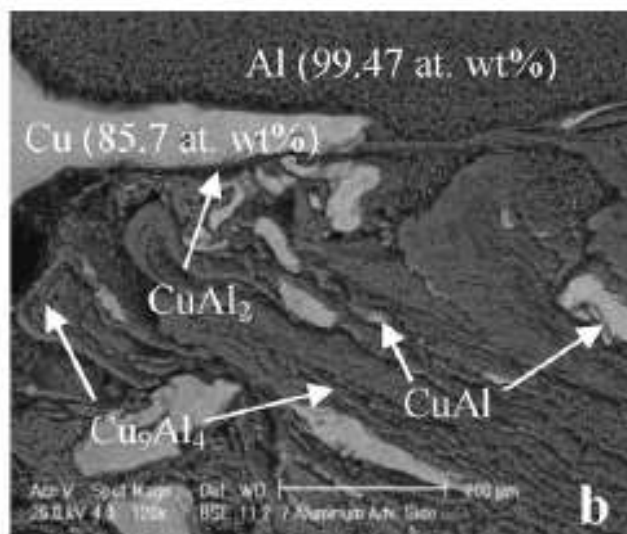
Εικ 1: SEM μικροδομή σε back scatter electron view της περιοχής συγκόλλησης [4]
