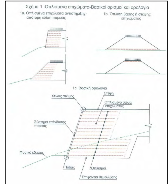
Εικόνα 1 - Οπλισμένες γαίες - τρόπος εφαρμογής
