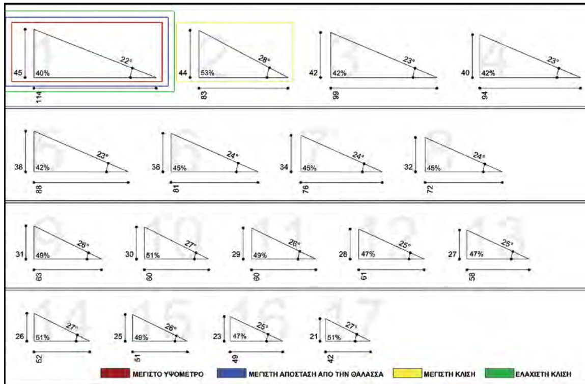
Εικόνα 15 - Τοπογραφικό 3 - Εγκάρσιες τομές
