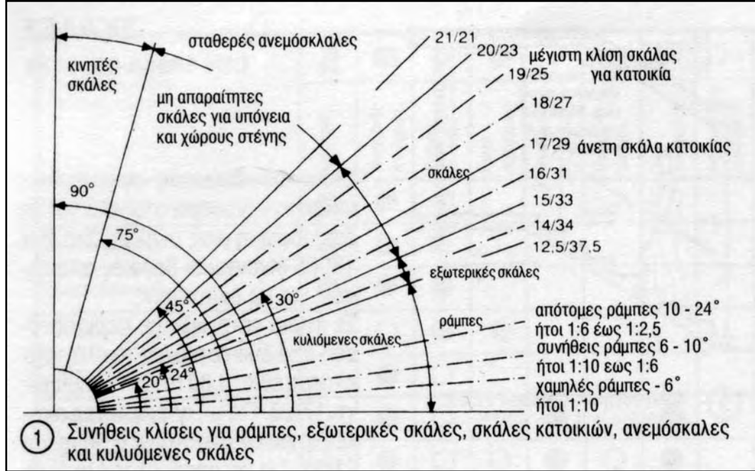
Εικόνα 17 - Πίνακας από το βιβλίο "Οικοδομική και αρχιτεκτονική σύνθεση", Neufert - όρια υποφερτής κλίσης
