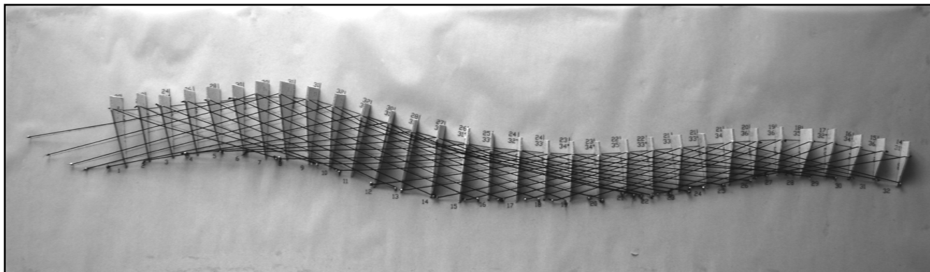
Εικόνα 29 - Τοπογραφικό 4 - κλίση των 9°, μακέτα τοπογραφικού με τον τρισδιάστατο κάρναβο.
