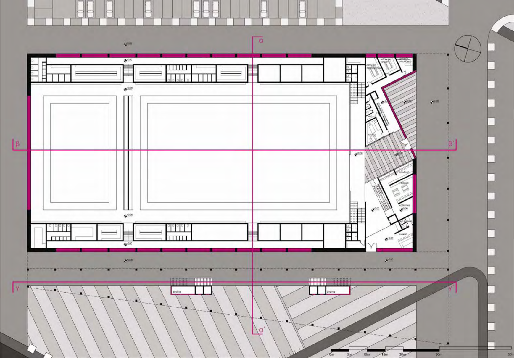
Εικόνα 53. Κάτωψη συγκροτήματος κολυμβητηρίου _ στάθμη +2.00m.
