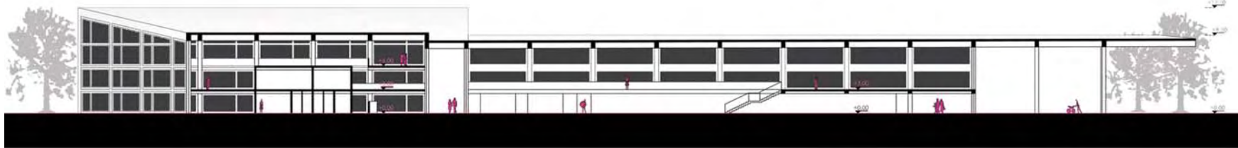
Εικόνα 64. Τομή συγκροτήματος ναυτικού ομίλου β-β'.
