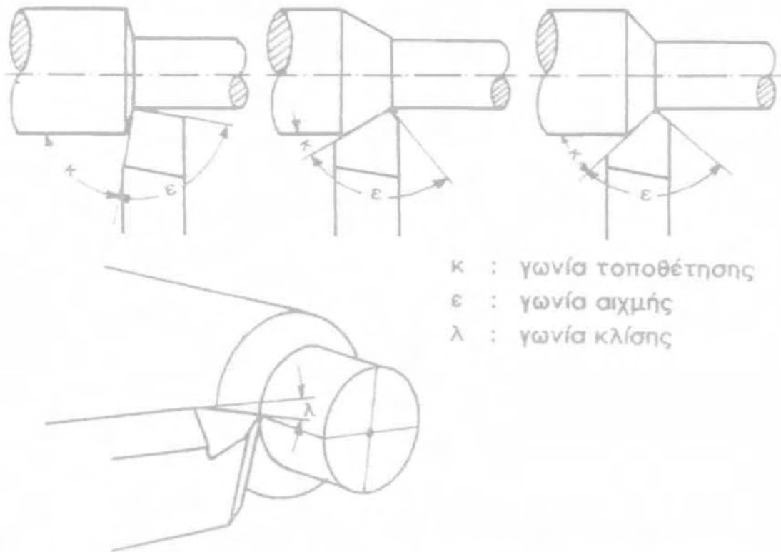
Σχήμα 2.7 Χαρακτηριστικές γωνίες τοποθέτησης κοπτικού εργαλείου τόρνευσης
