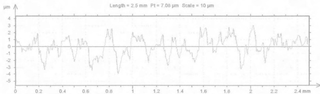
Διάγραμμα Π.17: Περίγραμμα επιφάνειας Ertacetal ( v=300\text{m/min} , f=0.05\text{mm/rev} )
