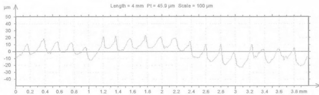
Διάγραμμα Π.47: Περιγράμμα επιφάνειας Ertacetal ( v=500\text{m/min} , f=0.20\text{mm/rev} )
