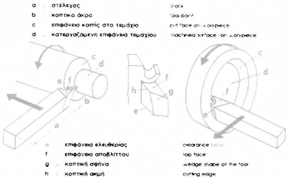
Σχήμα 2.4 Χαρακτηριστικές ακμές και επιφάνειες εργαλείου και τεμαχίου στην τórνευση
