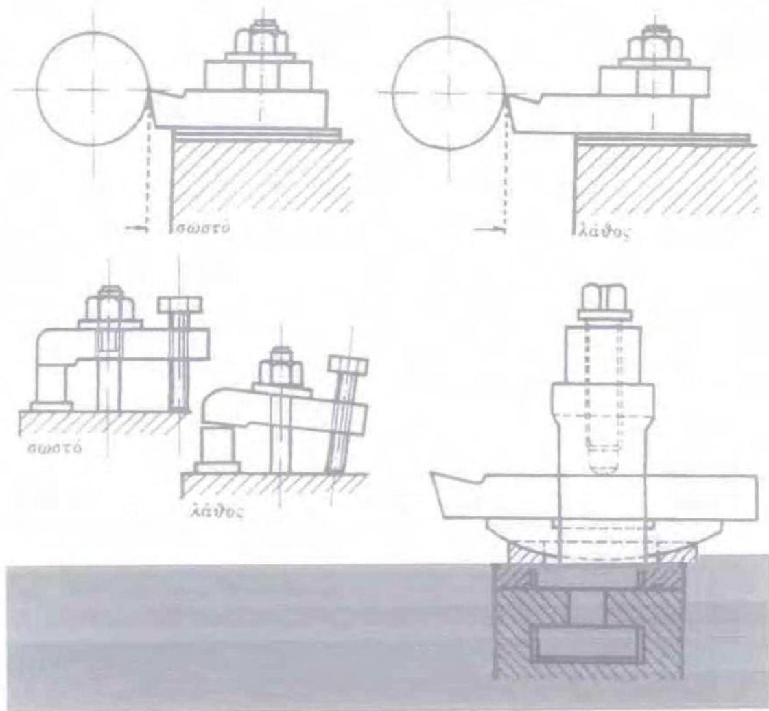
Σχήμα 2.2 Τρόπος συγκράτησης κοπτικών εργαλείων τórνευσης
