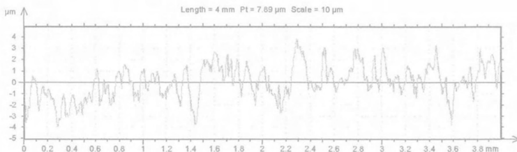
Διάγραμμα Π.37: Περιγραφή επιφάνειας Ertacetal ( v=200\text{m/min} , f=0.05\text{mm/rev} )
