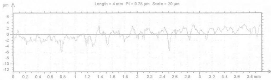
Διάγραμμα Π.46: Περιγράμμα επιφάνειας Ertacetal ( v=500\text{m/min} , f=0.10\text{mm/rev} )
