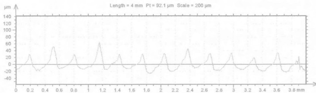
Διάγραμμα Π.48: Περιγράμμα επιφάνειας Ertacetal ( v=500\text{m/min} , f=0.32\text{mm/rev} )
