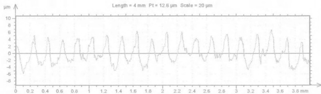
Διάγραμμα Π.27: Περιγράμμα επιφάνειας Ertacetal ( v=200\text{m/min} , f=0.20\text{mm/rev} )
