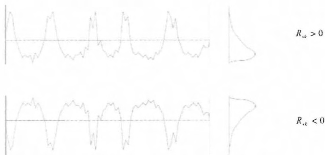
Σχήμα 2.17: Περιγράμματα επιφανειών με θετική και αρνητική λοξότητα
