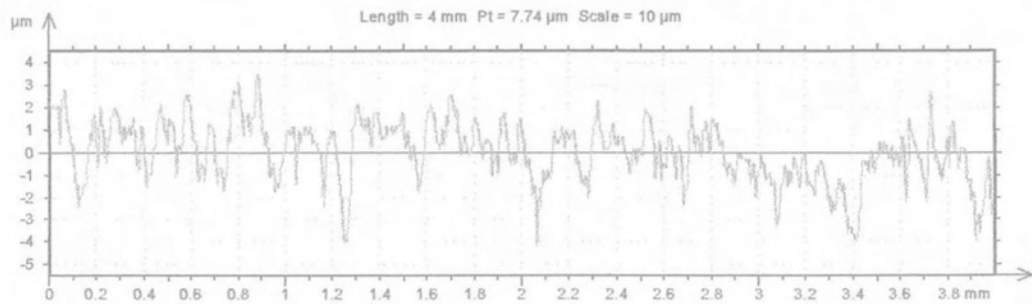
Διάγραμμα Π.25: Περιγράμμα επιφάνειας Ertacetal ( v=200\text{m/min} , f=0.05\text{mm/rev} )
