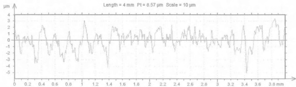
Διάγραμμα Π.41: Περιγράμμα επιφάνειας Ertacetal ( v=300\text{m/min} , f=0.05\text{mm/rev} )
