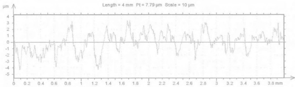
Διάγραμμα Π.25: Περιγράμμα επιφάνειας Ertacetal ( v=200\text{m/min} , f=0.05\text{mm/rev} )
