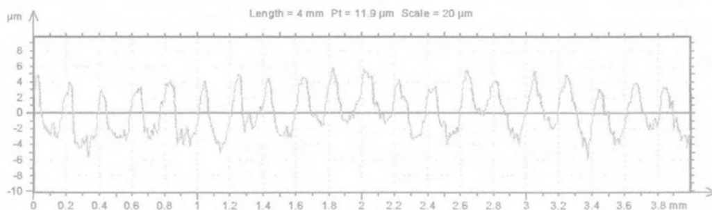
Διάγραμμα Π.38: Περιγραφή επιφάνειας Ertacetal ( v=200\text{m/min} , f=0.10\text{mm/rev} )
