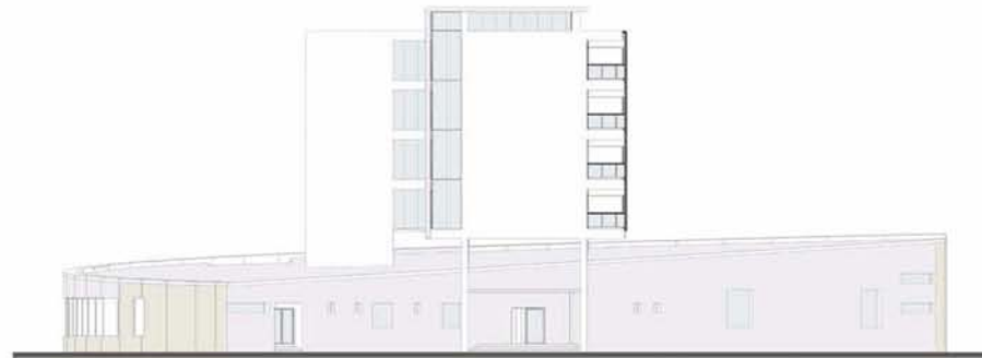
δυτική όψη
