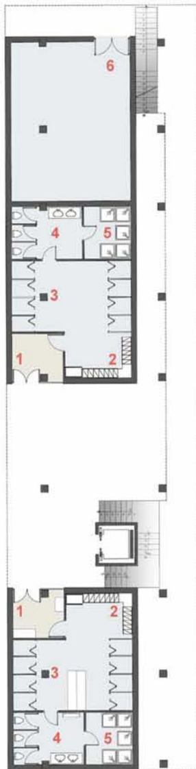
Αποδυτήρια παιδων-κορασίδων
