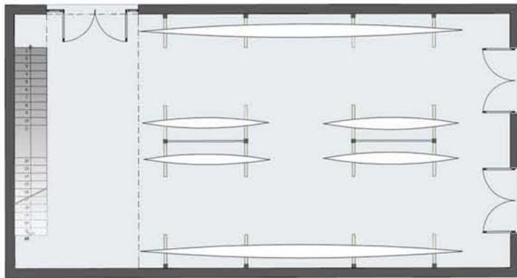
κάτοψη υπόστεγου σκαφών κωπηλασίας
