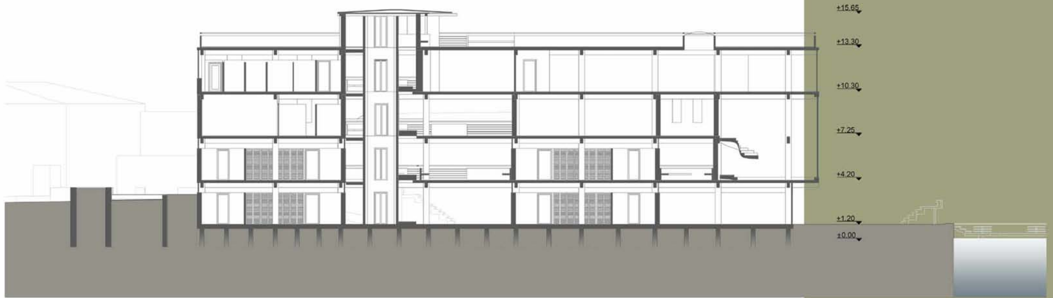
τομή ββ
