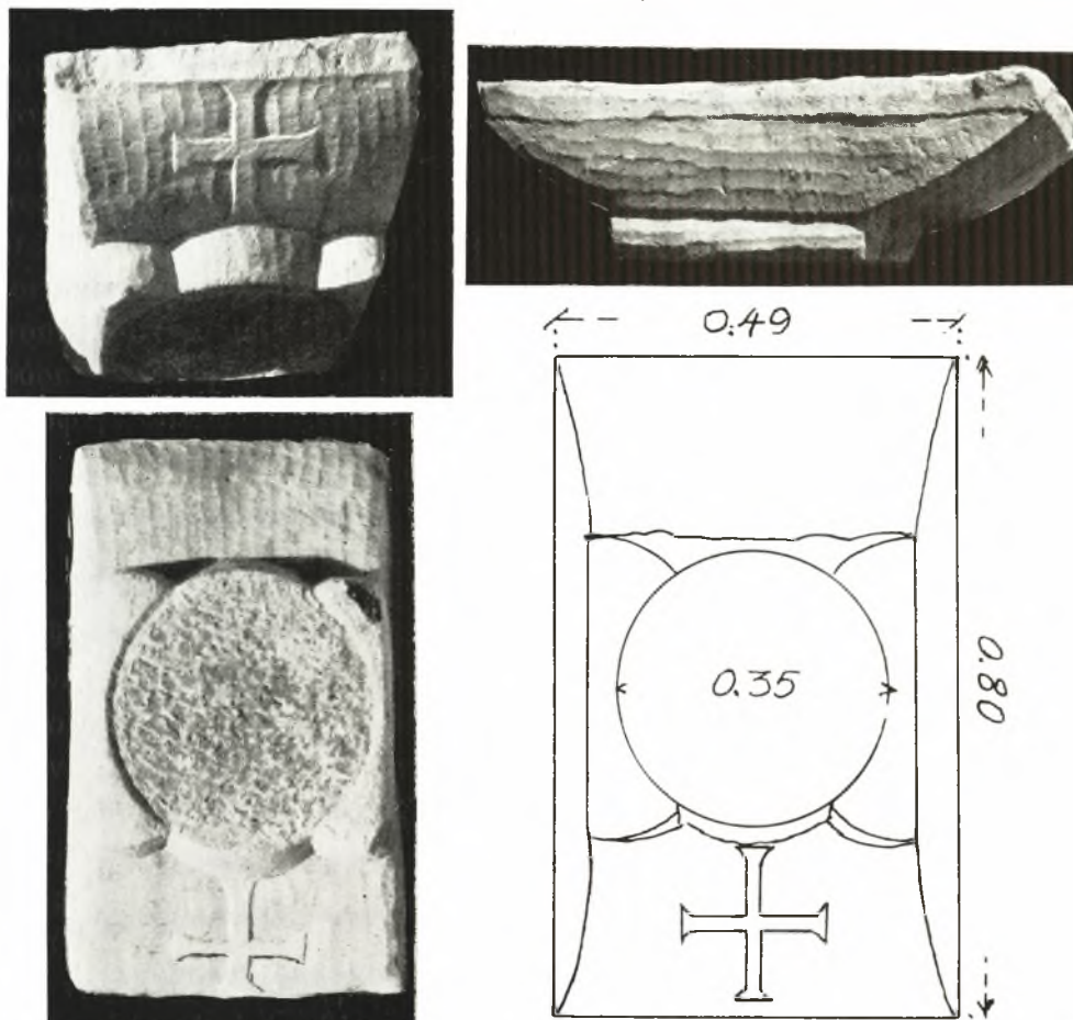
Εἰκ. 13. Κάτω: κατόψεις. Ἄνω: προσθία καὶ πλαγία ὄψεις τοῦ ἰωνικοῦ μετ' ἐπιθήματος κιονοκράνου.
