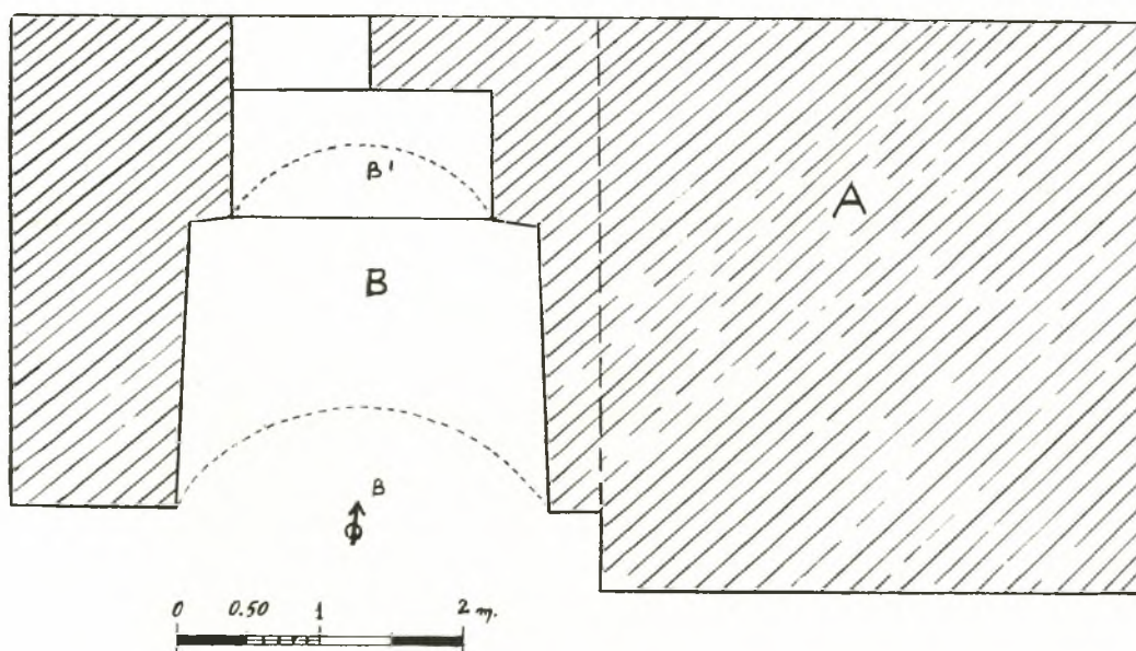
Εἰκ. 1. Κάτοψις βάσεως τῆς ῥωμαϊκῆς δεξαμενῆς.
