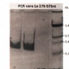
Εικόνα 70: Ηλεκτροφόρηση σε πήκτωμα ακρυλαμιδίου, του ενισχυμένου με PCR, τμήματος 273-573nt του γονιδίου core-1α του HCV για να ακολουθήσει καθαρισμός από πήκτωμα ακρυλαμιδίου TBE-PAGE 5%.
