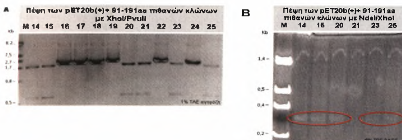
Εικόνα 51: Ηλεκτροφόρηση των πέψεων των πιθανών κλώνων 14-25 με τα ένζυμα XhoI/PvuII (A) σε 1% αγαρόζη για την εύρεση επιπλέον θετικών κλώνων pET20b(+) + 91-191aa του γονιδίου core του HCV. (B) Οι κλώνοι 14, 15, 20, 21, 23 και 25 στη συνέχεια πέπτονται με τα ένζυμα NdeI/XhoI. Όλοι εκτός από τον 21 εμφανίζουν ζώνες στο αναμενόμενο μέγεθος.
