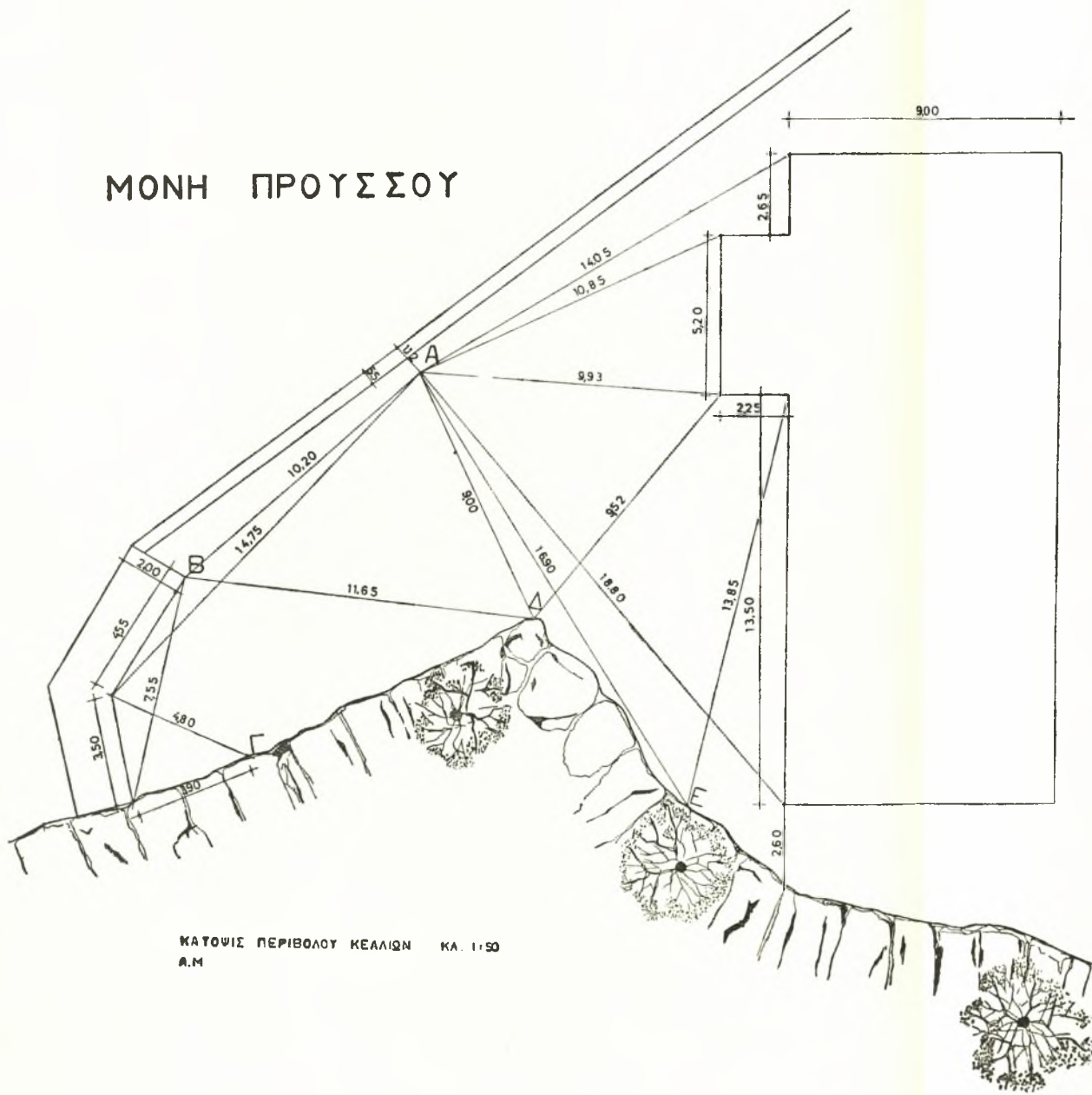
Σχεδ. 1. Κάτωγες τοῦ περιβόλου καὶ κελλιῶν τῆς Μονῆς Προῦσου
