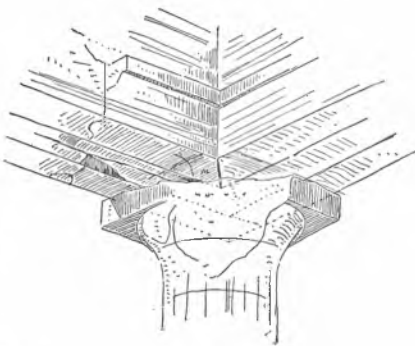
Σχῆμα 10. Βορειοδυτικὸς γωνιαῖος κίων τοῦ ὀπισθοδόμου. Ἐποψίς ἐκ τῶν ἐνδόν.
