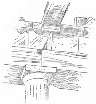
Σχῆμα 12. Δυτικὴ πλευρὰ τῆς περιστάσεως. Δεῦτερος κίων ἐκ μεσημβρίας.
