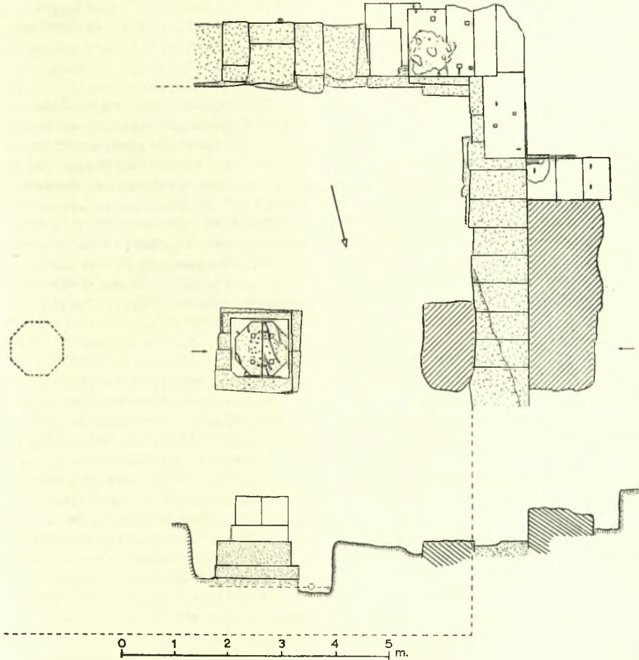
Σχέδ. 1. Κάτοψις καὶ τομὴ λειψάνων στοᾶς βορείου λιμένος Μυτιλήνης
