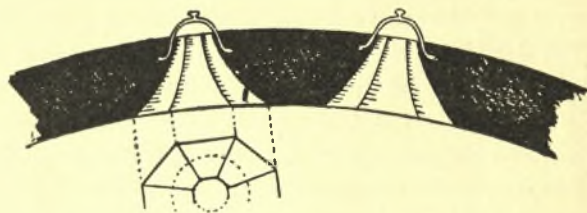
Εἰκ. 7. Διάταξις τῶν μικρῶν ὑαλίνων φωταγωγῶν εἰς τοὺς θόλους τῶν τουρκικῶν βαλανείων.
