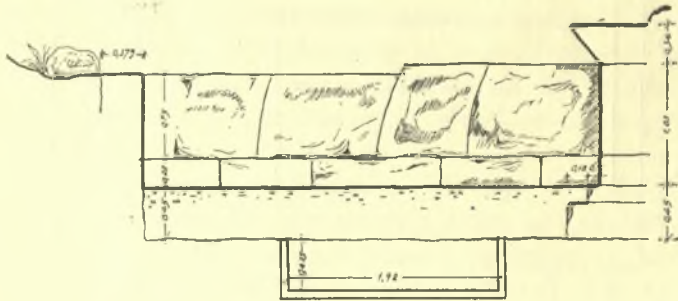
Εἰκ. 3. Β - Β'. Ἐγκαρσία τομὴ τοῦ ταφικοῦ κτίσματος.
