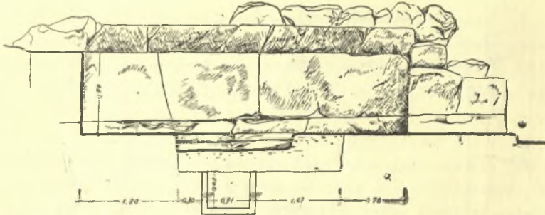
Εἰκ. 2. Α - Α'. Κατὰ μήκος τομὴ τοῦ ταφικοῦ κτίσματος.
