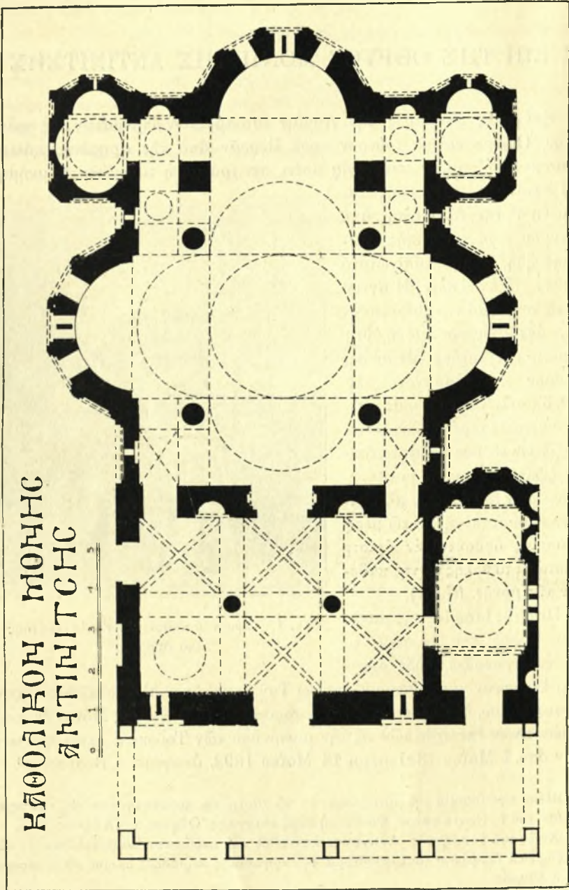
Είχ. 2. Κάτοψις τοῦ καθολικοῦ τῆς μονῆς Ἀγνίτισης.
