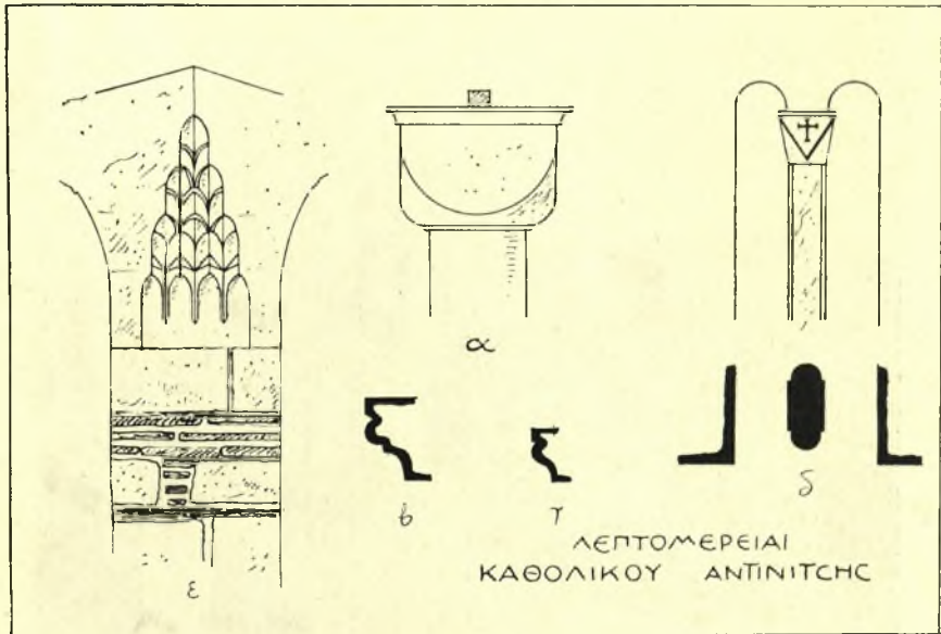
Εἰκ. 4. Λεπτομέρειαι τοῦ καθολικοῦ τῆς Ἀντινίτσης: α κιονόκρανον, β, γ τομαὶ κοσμητῶν, δ παράθυρον ἱεροῦ, ε σταλακτιτοειδῆς διαμόρφωσις τῆς γωνίας τῶν παρεκκλησίων.
