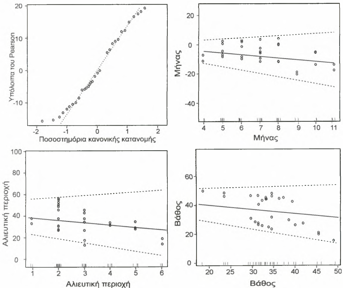
Εικόνα 3.4. Ανάλυση υπολοίπων και κύριες επιδράσεις του μήνα αλίευσης, της αλιευτικής περιοχής και του βάθους αλίευσης του μοντέλου που εφαρμόστηκε στις εκφορτώσεις του σαφριδιού.
