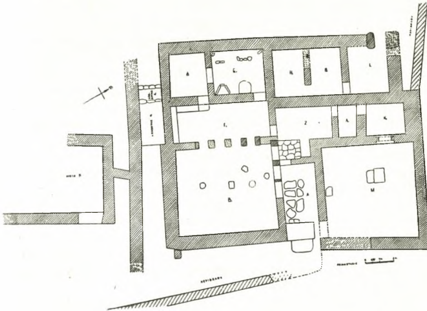
Εἰκ. 1. Κάτοψις μεσομινωικῆς οἰκίας Α Ρίζας 'Αχλαδιῶν Σητείας.
