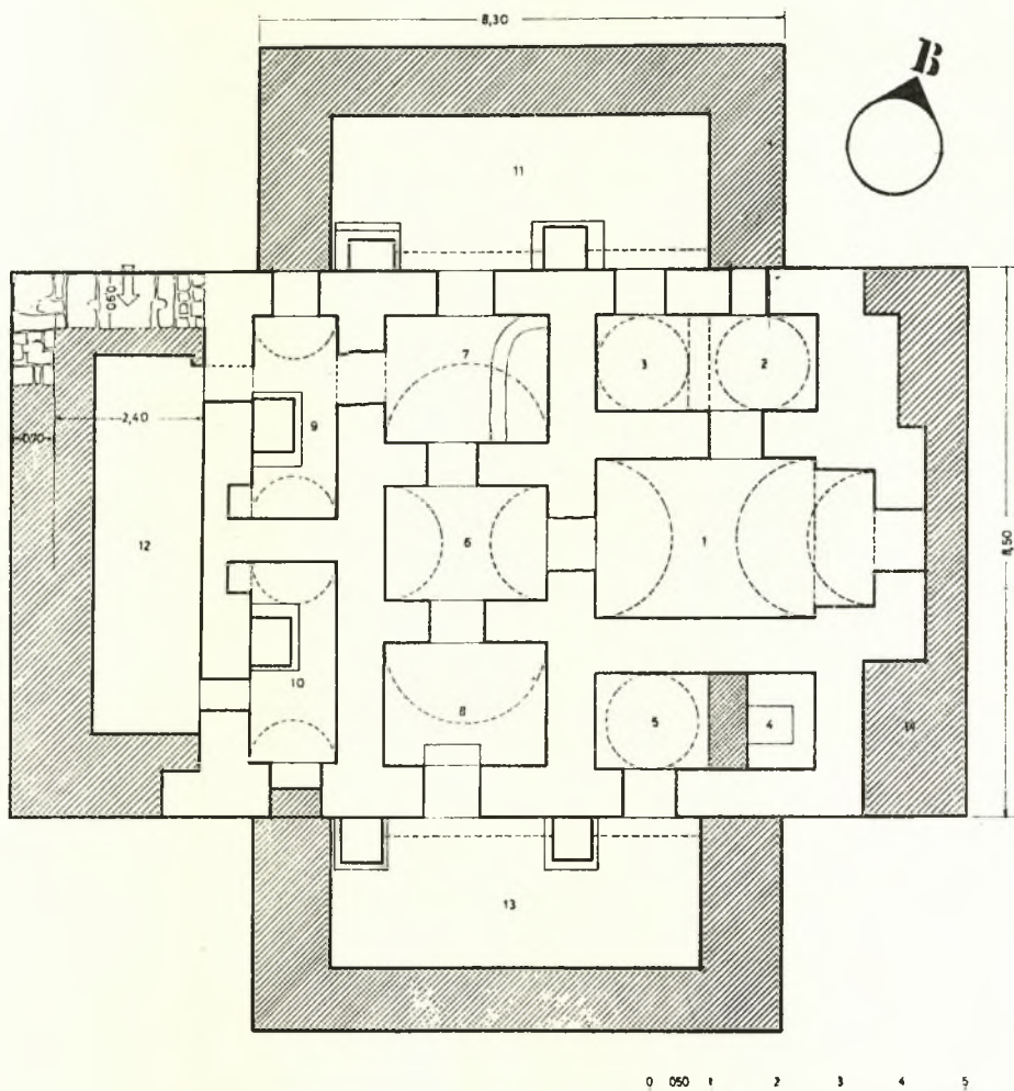
Σχέδ. 1. Διώροφον κτηριακὸν συγκρότημα εἰς θέσιν Πύργος. Κάτωψιν ἰσογείου
