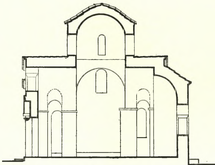
Σχ. 6. Σχηματάρι. Ναὸς Ἁγίου Ἰωάννου. Τομή κατὰ μήκος
