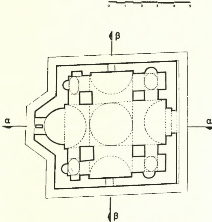
Σχέδ. 5. Σχηματάρι. Ναὸς Ἁγίου Ἰωάννου. Κάτοψις
