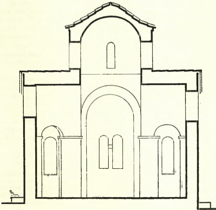
Σχέδ. 7. Σχηματᾶρι. Ναὸς Ἁγίου Ἰωάννου. Τομὴ κατὰ πλάτος
