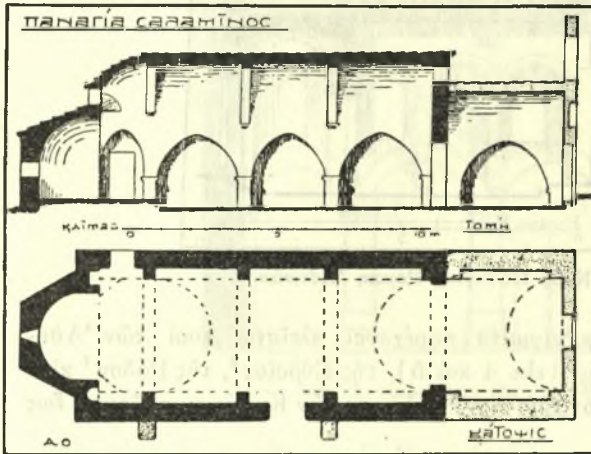
Εἰκ. 4. Ναὸς Παναγίας Σαλαμίνος. Κάτοψις καὶ τομῆ.
