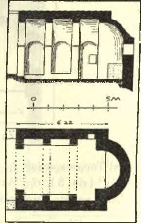
Εἰκ. 5. Ναὸς Ἁγ. Δημητρίου εἰς Ἄνω Σοῦλι.
