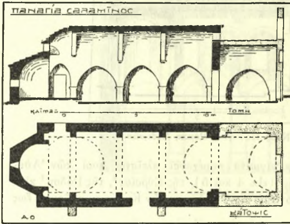
Εἰκ. 4. Ναὸς Παναγίας Σαλαμίνος. Κάτοψις καὶ τομῆ.
