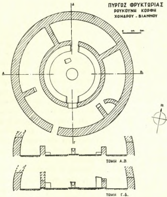
Εἰκ. 3. Κάτοψις καὶ κατακόρυφοι τομαὶ πύργου φρυκτωρίας Ρουκούνη Χόνδρου Βιάννου.
