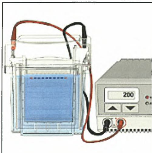
Εικόνα 6: Συσκευή ηλεκτροφόρησης.
