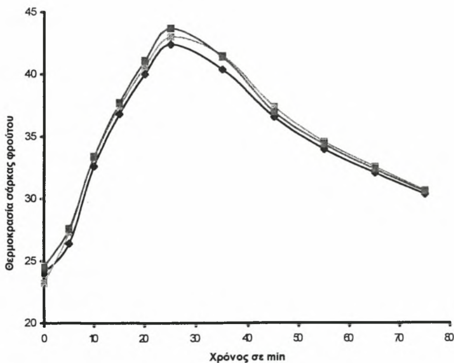
Σχεδ.1. Θερμοκρασία της σάρκας του φρούτου κατά τη διάρκεια και μετά τη θέρμανση με νερό 46^\circ\text{C}
