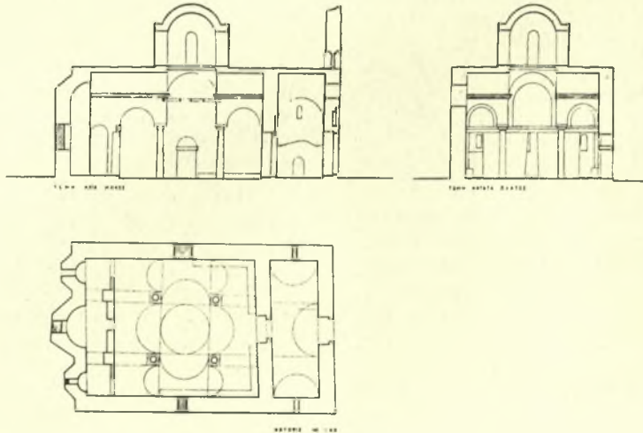
Σχέδ. 1. Ἅγιος Ἰωάννης Κέριας. Κάτοψεις καὶ τομαί
