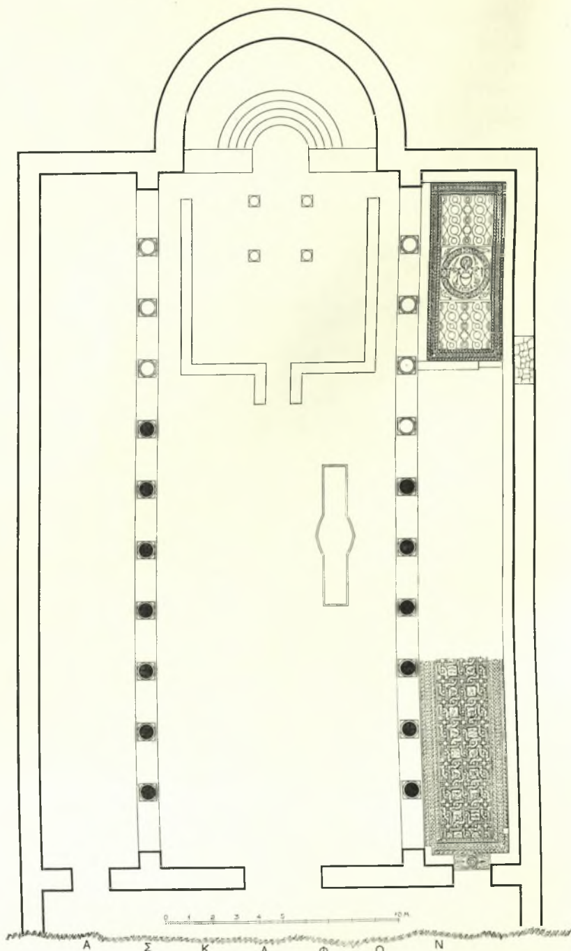
Είκ. 1. Κάτοψις τῆς βασιλικῆς Α μετὰ τὴν ἀνασκαφὴν τοῦ 1967.
