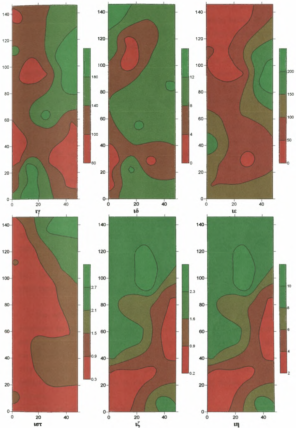
(γ) ppm Ca, (ιδ) ppm Fe, (ε) ppm Na, (ιστ) ppm Zn, (ιζ) ppm Cu, (ιη) ppm Mn Σχήμα 5.8. Χάρτες εδαφικών παραμέτρων για βάθος 30-60 εκ.
