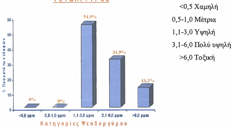
Σχήμα 3.9. Διαθεσιμότητα Ψευδαργύρου
