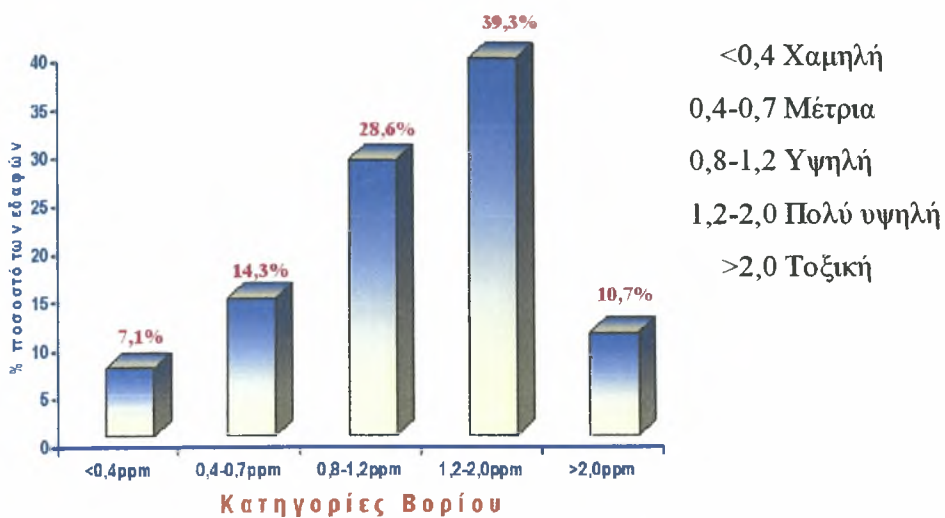
Σχήμα 3.8. Διαθεσιμότητα Βορίου
