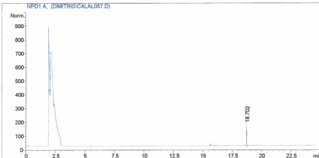
Σχήμα 7. Χρωματογράφημα ενός προτύπου διαλύματος alachlor συγκέντρωσης 20 mg/L
