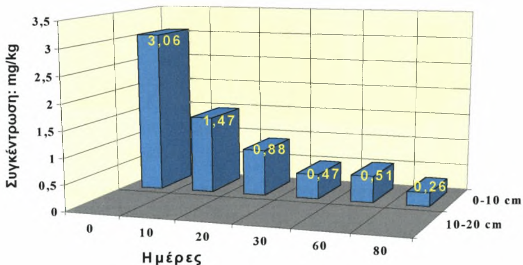
Σχήμα 10. Μεταβολή των υπολειμμάτων του alachlor στο έδαφος σε σχέση με το χρόνο στο 2 ο πείραμα.
