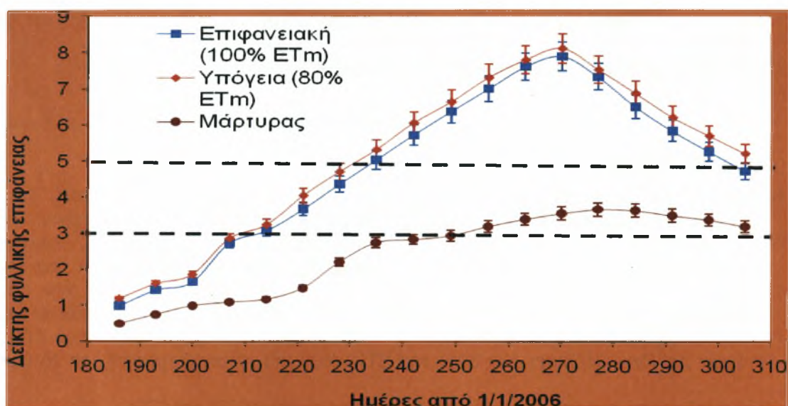
Διάγραμμα 5.6 Η εξέλιξη του δείκτη φυλλικής επιφάνειας L.A.I.
