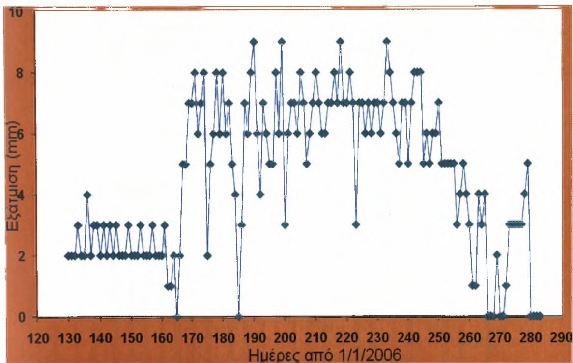
Διάγραμμα 5.2. Διακύμανση της εξάτμισης κατά τη διάρκεια του πειράματος
