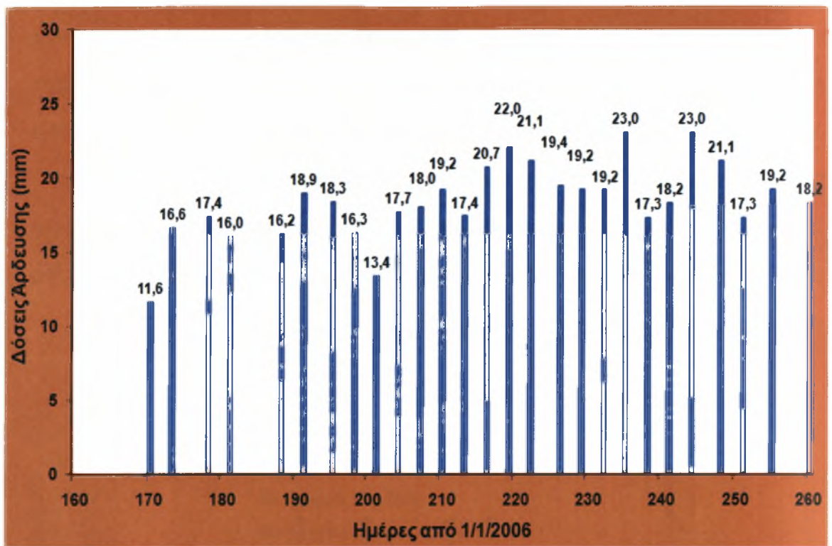
Διάγραμμα 5.3. Δόσεις άρδευσης στην επιφανειακή στάγδην στο 100% της ETm.
