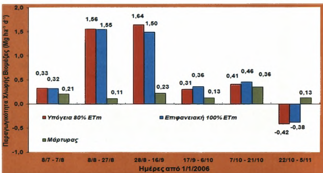
Διάγραμμα 5.8 Παραγωγικότητα σε χλωρή βιομάζα για όλες τις μεταχειρίσεις
