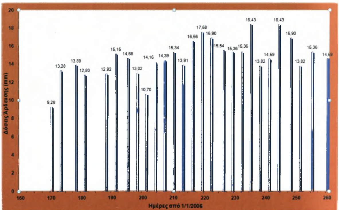
Διάγραμμα 5.4. Δόσεις άρδευσης στην υπόγεια στάγδην στο 80% της ETm
