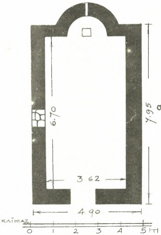
(Εἰκ. 2) Κάτοψις τοῦ ναοῦ τῆς Δουπιάνης 5) .
