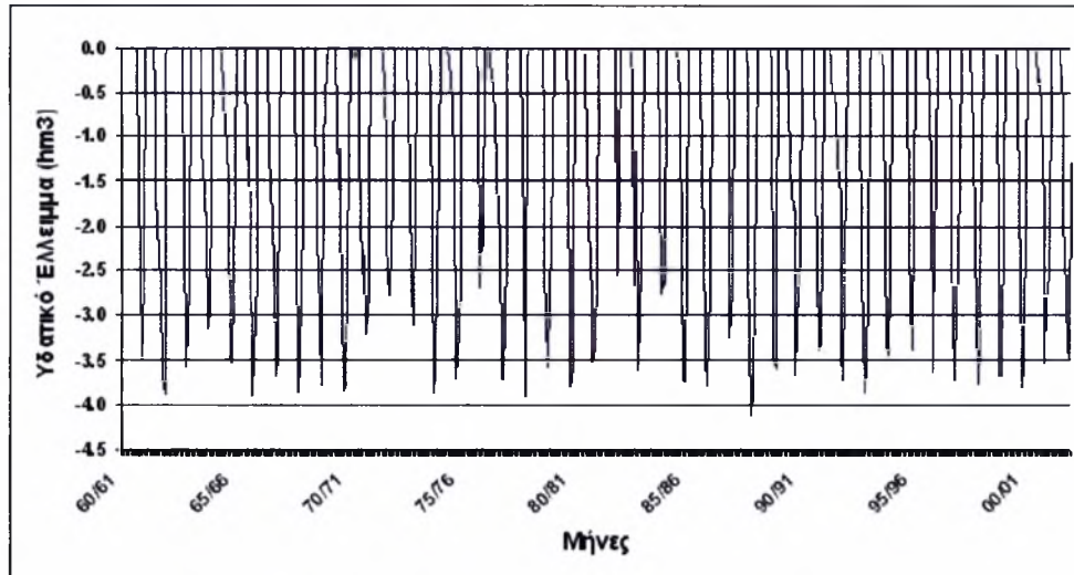
Σχήμα 6.2.11 Μηνιαίο υδατικό ισοζύγιο του ταμιευτήρα Κλινοβού
