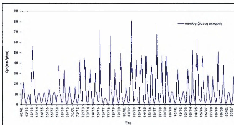
Σχήμα 4.3.3. Υπολογισμένες τιμές Q_c της λεκάνης απορροής Μαυρομάτη για την υδρολογική περίοδο Οκτώβριος 1960 – Σεπτέμβριος 2002.
