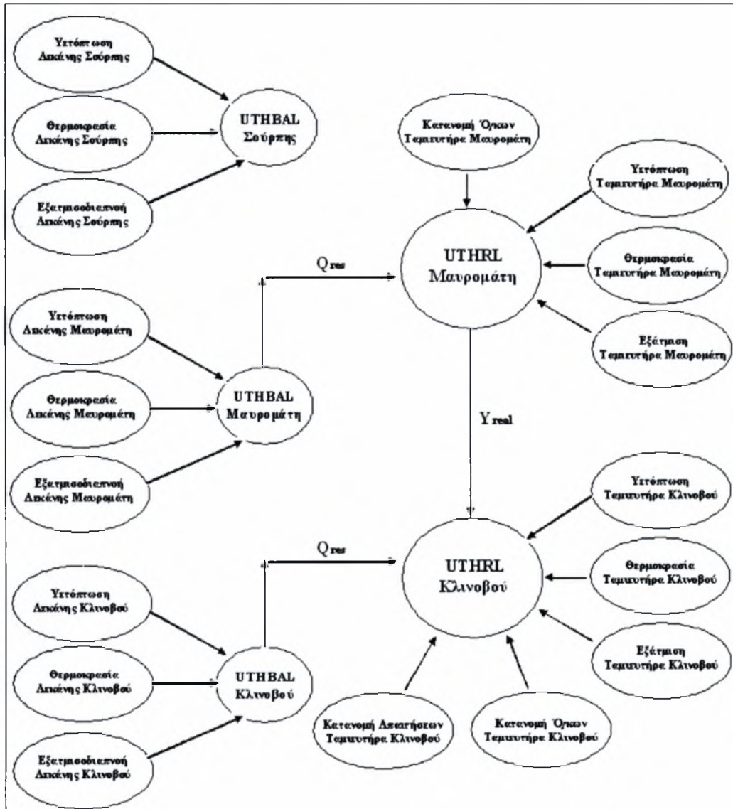
Σχήμα 7.11.1. Διάγραμμα ροής στοχαστικής προσομοίωσης υδατικού συστήματος υδρολογικής λεκάνης Σούρπης
