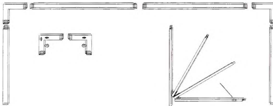
ΣΥΝΑΡΜΟΛΟΓΗΣΗ ΤΟΥ ΣΚΕΛΕΤΟΥ ΤΗΣ ΤΕΝΤΑΣ
