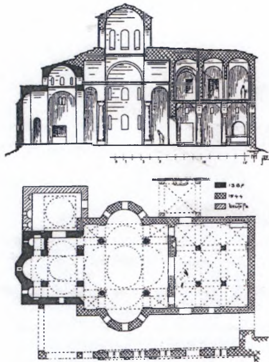
Εικ. 8 Μετέωρα, Μονή Μεγάλου Μετεώρου, παλαιό και νέο καθολικό. Κάτοψη και τομή (Σοφιανός 1990, εικ. στη σ. 103).
