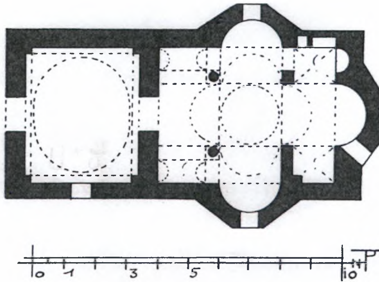
Εικ. 1 Μετέωρα, Μονή Ρουσάνου, καθολικό. Κάτοψη (Σοφιανός 1990, εικ. στη σ. 78).
