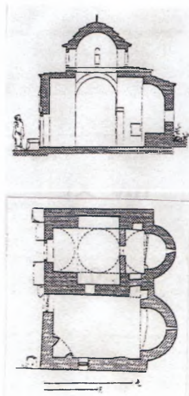
Εικ. 32 Χαλιδού Αττικής, Άγιος Νικόλαος. Κάτοψη και τομή (Μπούρας, Μπούρα 2002, εικ. 394).
