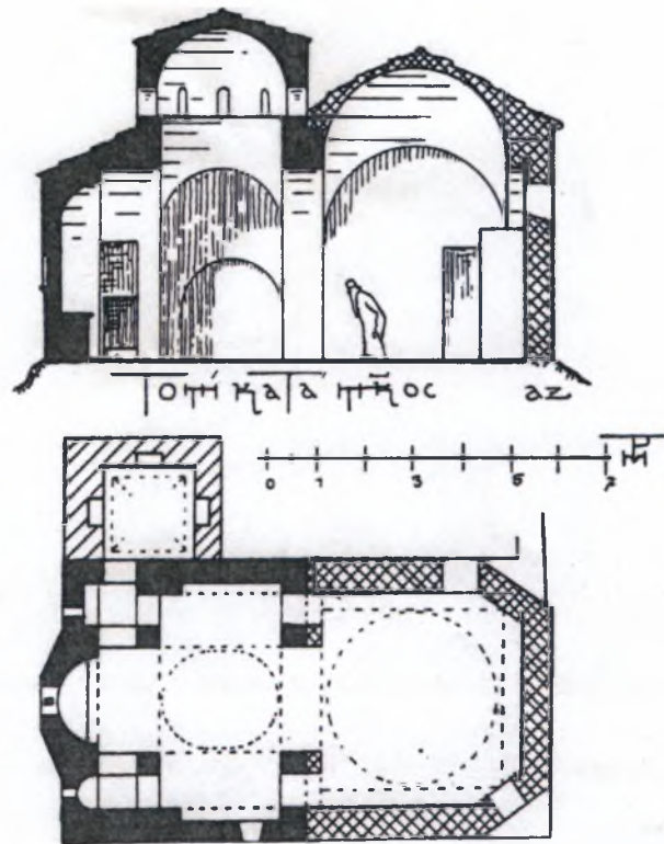
Εικ. 20 Μετέωρα, Μονή Αγ. Τριάδας, καθολικό. Κάτοψη και τομή (Σοφιανός 1990, εικ. στη σ. 90).
