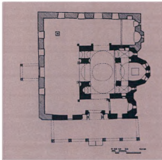
Εικ. 30 Θεσσαλονίκη, Μονή Βλατάδων, καθολικό. Κάτοψη (Κουρκουτίδου-Νικολαΐδου, Τούρτα 1997, εικ. 113).
