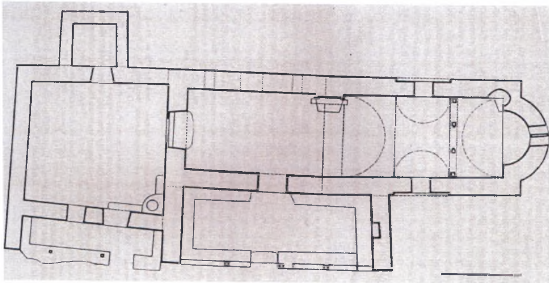
Εικ. 34 Αχλαδοχώρι Τρικάλων, Κοίμηση της Θεοτόκου. Κάτοψη (Νικονάνος 1997, σχ. 17).
