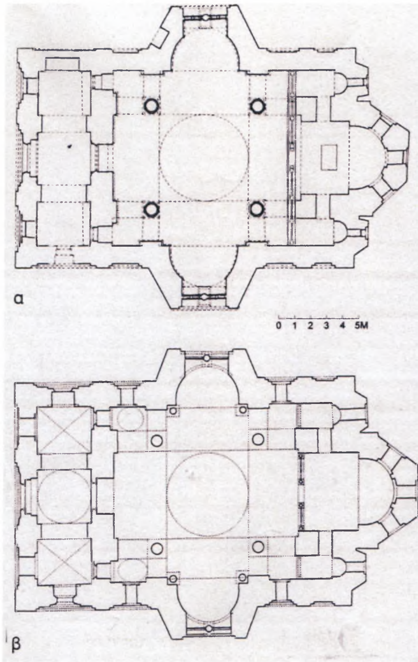
Εικ. 26. α. Άγιον Όρος, καθολικό Μονής Βατοπεδίου. Κάτοψη β. Άγιον Όρος, καθολικό Μονής Ιβήρων. Κάτοψη (Μαμαλούκος 2003, εικ. 4 α.β.).
