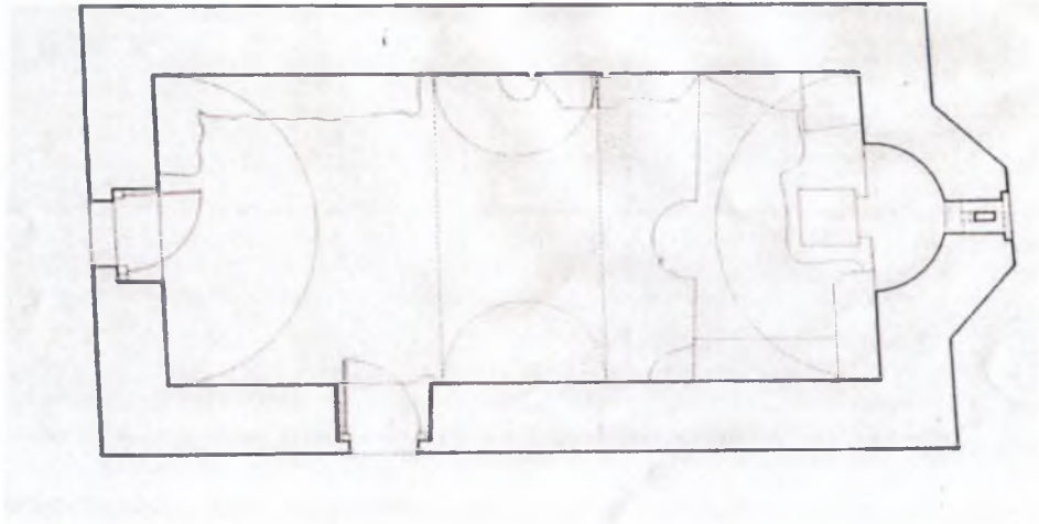
Εικ. 33 Λεοντάρι Αρκαδίας, Άγιος Αθανάσιος. Κάτοψη (Albani 1989, πίν. 1).
