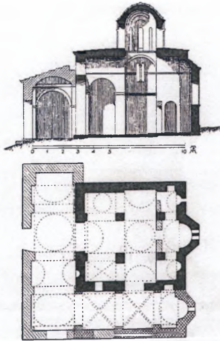
Εικ. 29 Αθήνα, Όμορφη Εκκλησιά. Κάτοψη και τομή (Γκιοιές 1992, εικ. 80).
