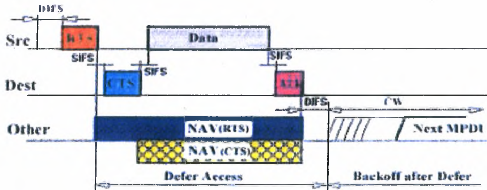
Εικόνα 11: Η διαδικασία CSMA/CA και Ack (αυτή που ακολουθεί το 802.11)
