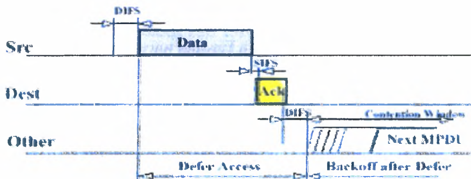
Εικόνα 10: Η διαδικασία CSMA και Ack
