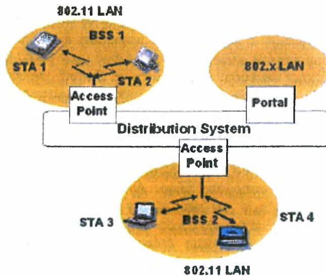
Εικόνα 9: Εκτεταμένο Σύνολο Υπηρεσιών (ESS)
