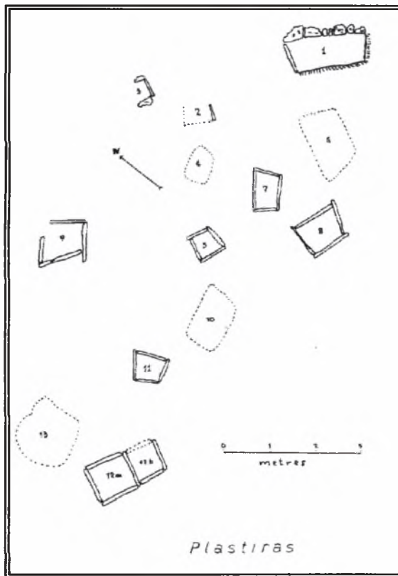
Εικ. 29 - Τοπογραφικό σχεδιάγραμμα των τάφων του νεκροταφείου Πλαστήρας της Νάξου (Doumas 1977, 33).
