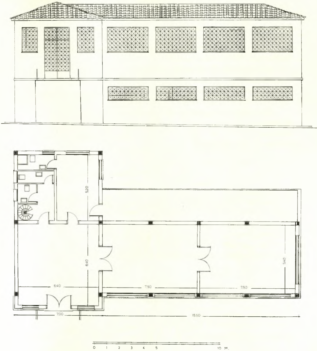
Εἰκ. 1. Κάτοψις καὶ πρόσοψις τοῦ διωρόφου νέου μουσείου (ἀρχαίας Μεσσήνης).
