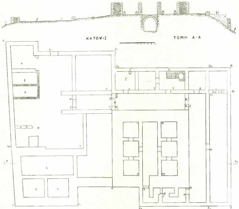
Εἰκ. 1. Κάτωψις καὶ τομὴ τοῦ Νεοκωμαντείου τῆς Ἐφύρας.
