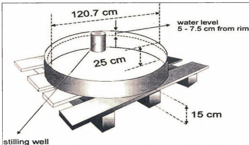
Εικόνα 2.16 Διαγραμματική απεικόνιση του εξατμισιμέτρου
