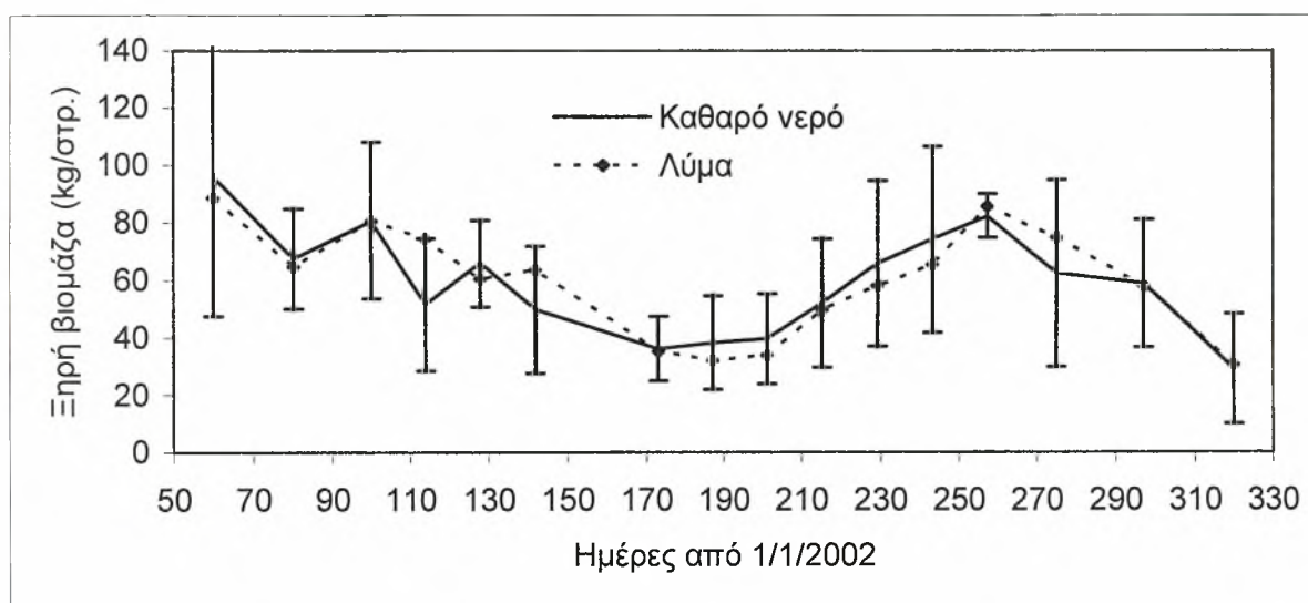
Σχήμα 3.5 Διακύμανση της απόδοσης σε ξηρή βιομάζα του χλοοτάπητα. Οι κάθετες ράβδοι αναφέρονται σε LSD_{p=0,05} .
