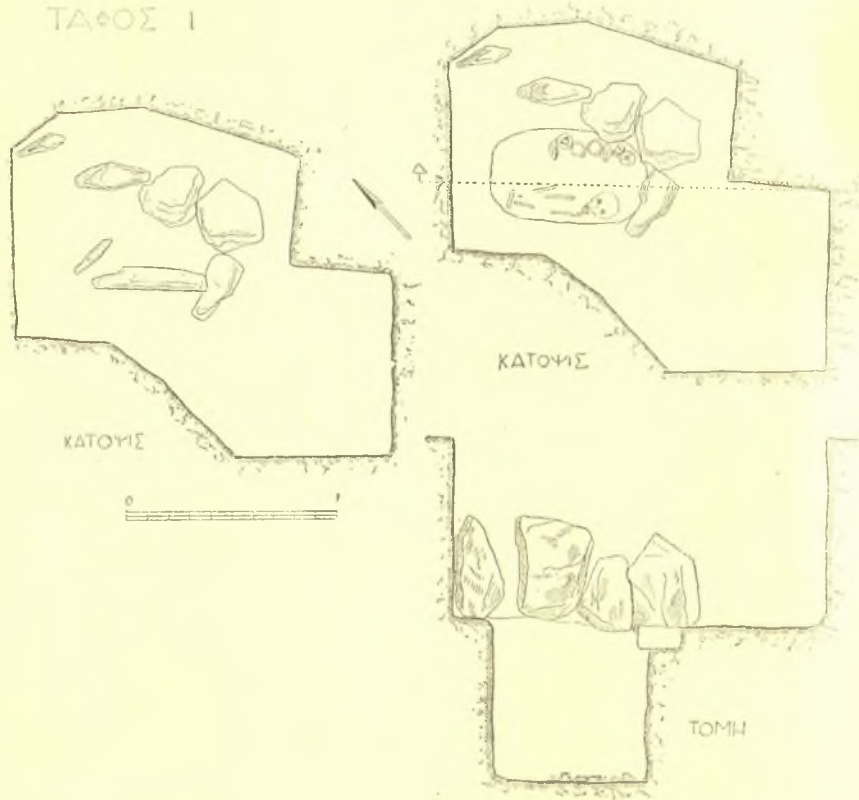
Εἰκ. 3. Κάτοψις καὶ τομή λακκοειδοῦς ταφῆς.
