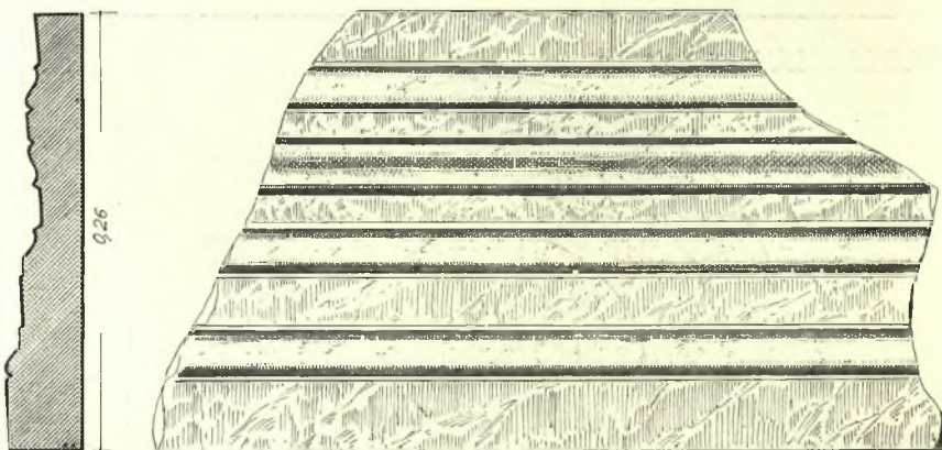
Εἰκ. 9. Τμήμα τοῦ μαρμαρίνου τοιχοβάτου (τομὴ καὶ ὀρθὴ προβολή).
