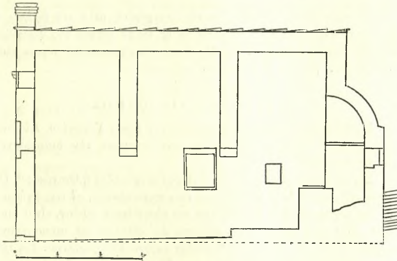
Σχεδ. 3. -- Ἅγιος Γεώργιος Ἄρτου Ρεθύμνης. Τομή κατὰ μῆκος.
