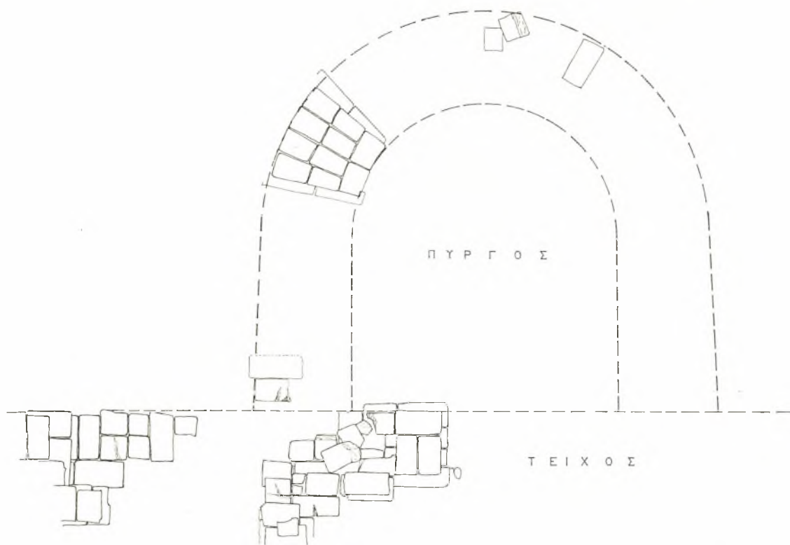
Εἰκ. 1. Συμπεληρωμένη κάτοψις θεμελιώσεως τοῦ παρὰ τὸν λιμένα τῆς Ἀκανδιᾶς Πύργου τῆς Ρόδου.
