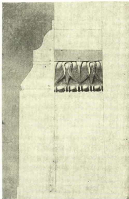
Εἰκ. 16. Τομὴ τοῦ ἐπίκρανου τῆς παραστάδος μετὰ τοῦ ἐπὶ τοῦ λεσβίου κυματίου κοσμήματος κατὰ τὴν Exped. Scient. de Morée.
