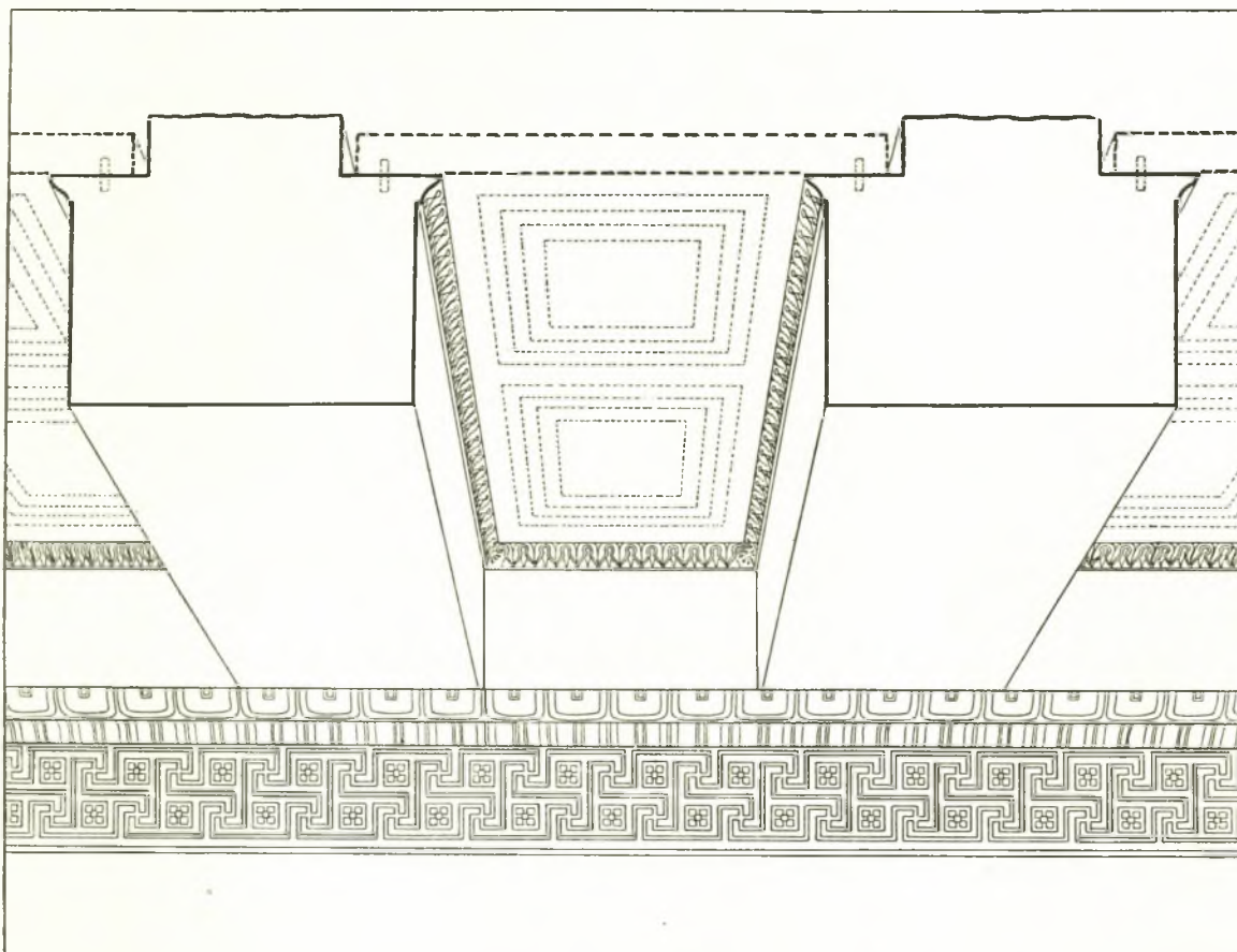
Εἰκ. 13. Προοπτικὴ ἀναπαράστασις τμήματος τῆς ὀροφῆς τοῦ περοῦ μετὰ τοῦ κοσμήματος τοῦ κάτωθεν αὐτῆς θράνου. Τὰ ὑποθετικὰ φατνώματα δι' ἐστιγμένων γραμμῶν.
