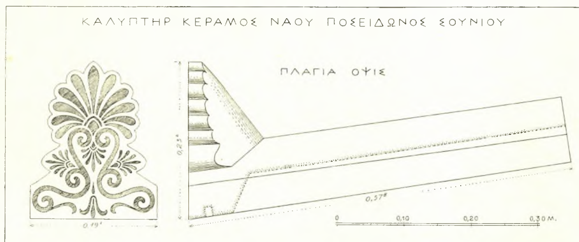
Εἰκ. 6. Ἡγεμῶν καλυπτὴρ κέραμος τοῦ ἐν Σουνίῳ ναοῦ τοῦ Ποσειδῶνος: ἄριστερᾷ πρόσοψις ἐν ἀναπαραστάσει, δεξιᾷ πλαγία ὄψις.
