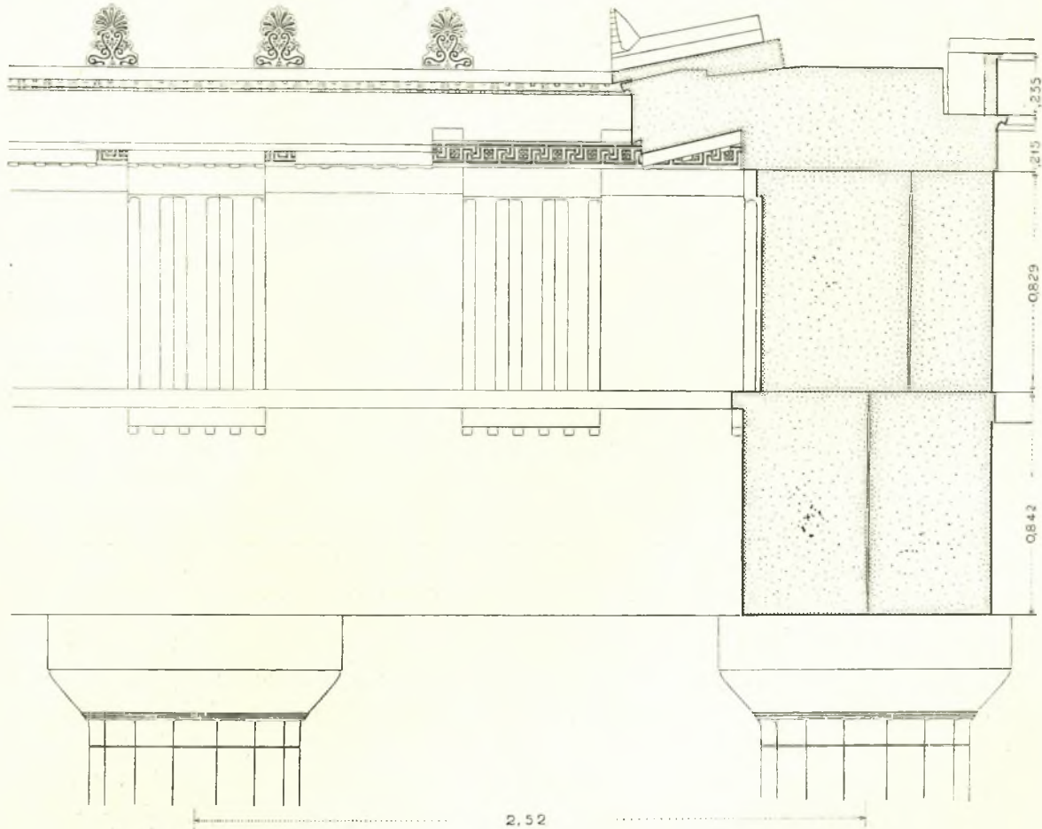
Εἰκ. 7. Τμήμα τῆς προσόψεως τῶν μακρῶν πλευρῶν τοῦ ναοῦ τοῦ Ποσειδῶνος δεικνύον τὸν κατὰ τὴν ρίζαν τοῦ γείσου γραπτὸν μαϊάνδρον.
