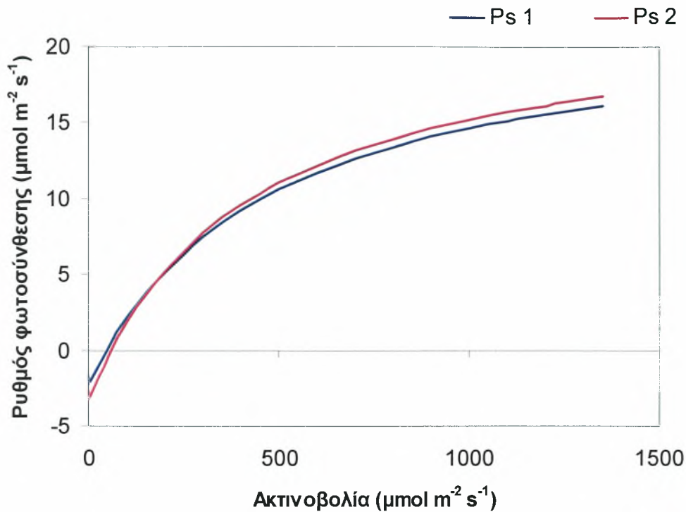
Σχήμα 5.6. Υπολογισμένες τιμές φωτοσύνθεσης συναρτήσεϊ της ακτινοβολίας, όπου Ps1: υπολογισμένες τιμές της φωτοσύνθεσης κατά τη μέτρηση στις 21 Απριλίου υπό την κάλυψη του UV5 υλικού στο UV5 θερμοκήπιο, Ps 2: υπολογισμένες τιμές της φωτοσύνθεσης κατά τη μέτρηση στις 27 Μαΐου υπό την κάλυψη του UV5 υλικού στο UV0 θερμοκήπιο.
