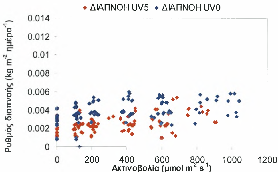
Σχήμα 4.5. Διαπνοή συναρτήσει της ακτινοβολίας κατά την περίοδο από 21 έως 22 Απριλίου.
