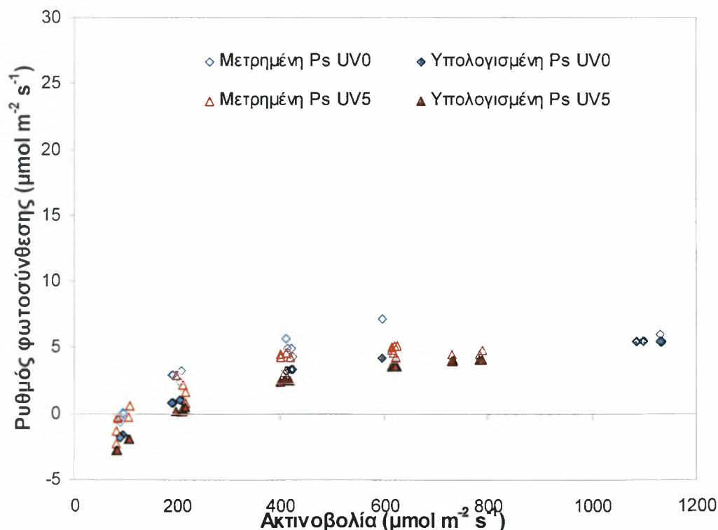
Σχήμα 4.4. Φωτοσύνθεση συναρτήσεϊ του ρυθμού ακτινοβολίας κατά την περίοδο 24 έως 29 Ιουνίου.
